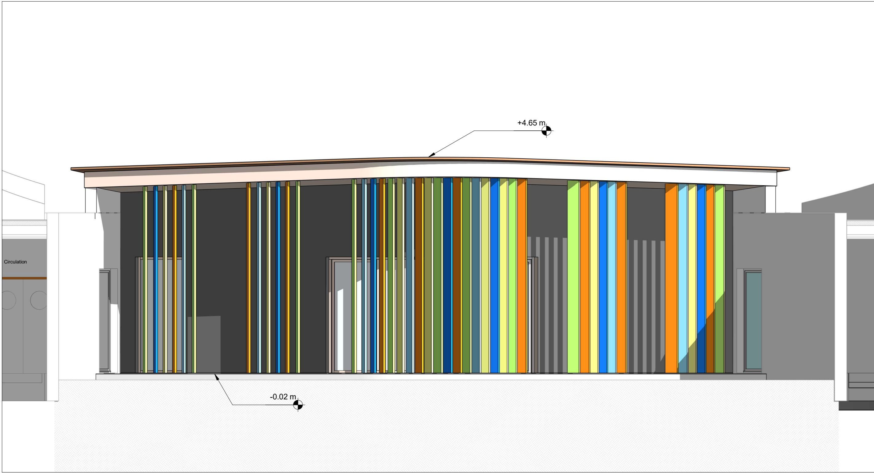
1 Elévation sud de la nouvelle classe Ech 1 : 50
