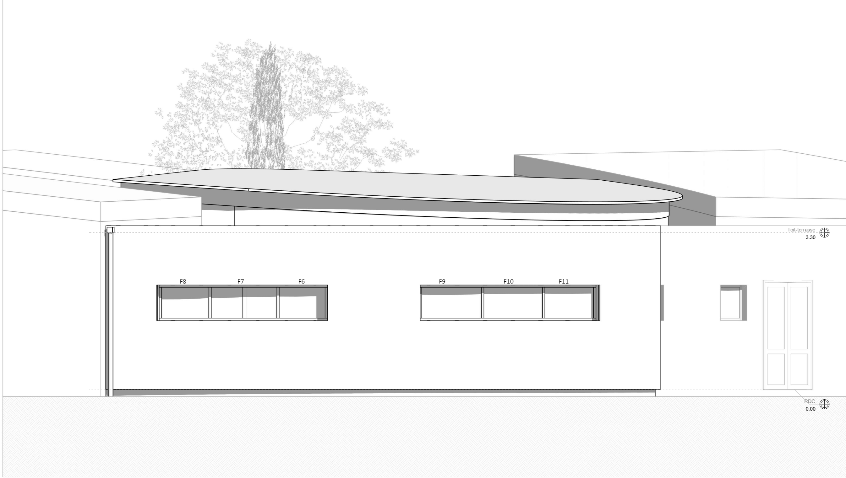
1 Elévation Nord des nouveaux sanitaires Ech 1 : 50
