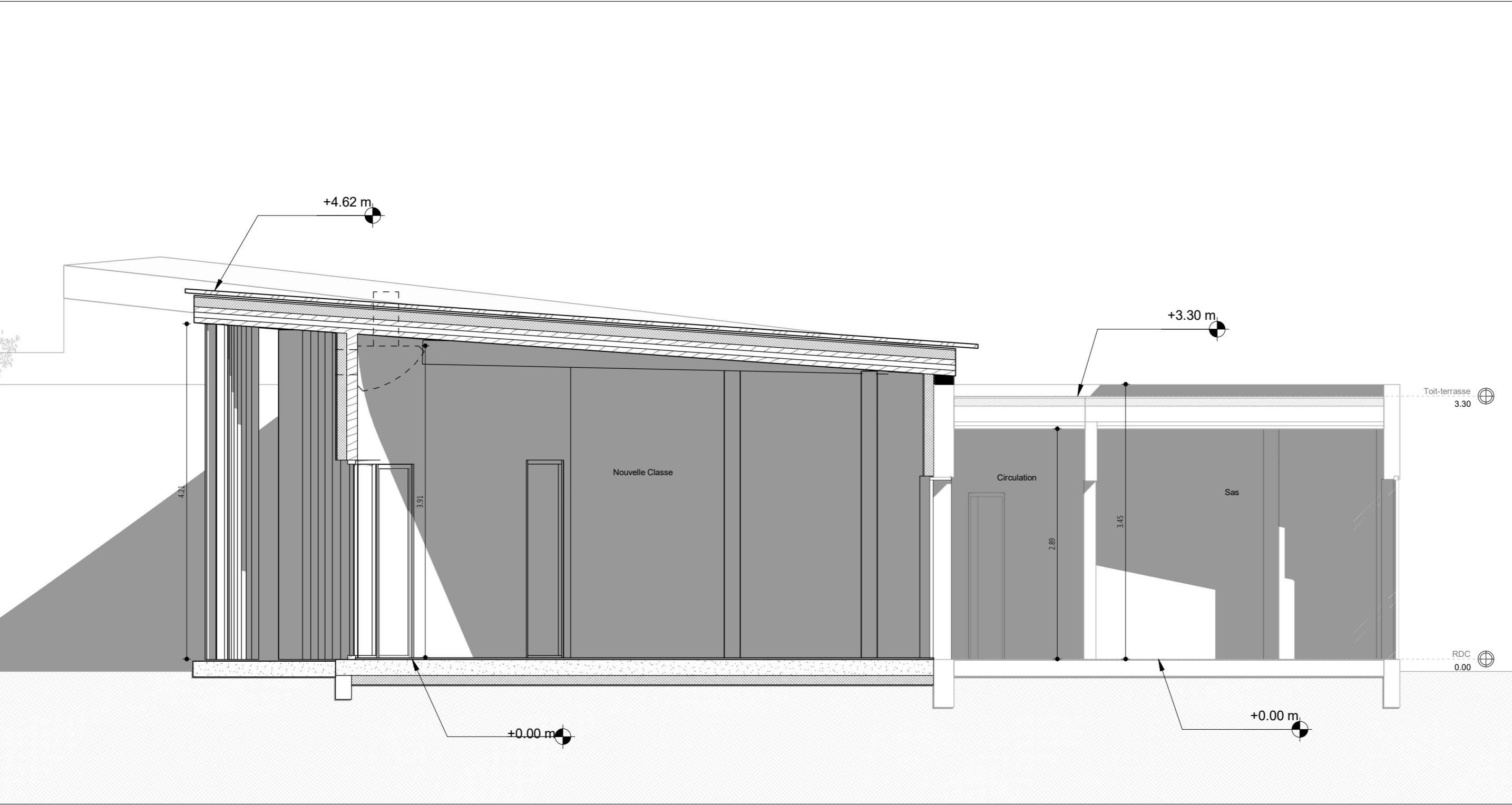
1 Coupe transversale sur la nouvelle Classe Ech 1 : 50
