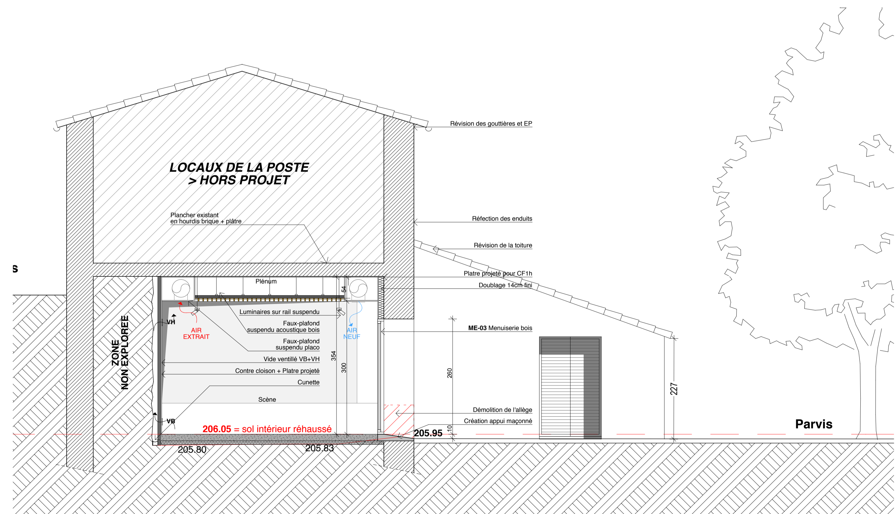
COUPE CC'
