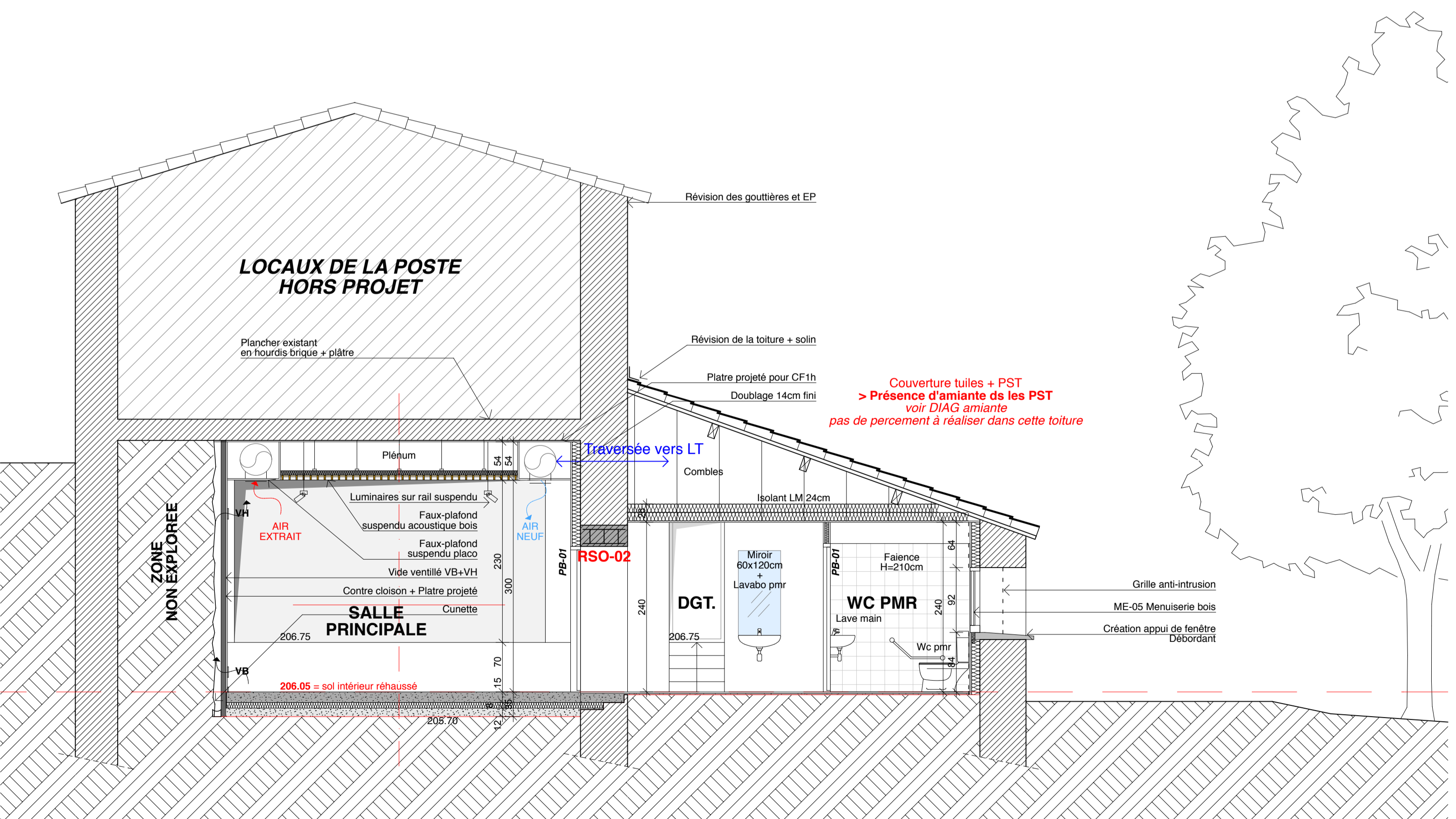
COUPE BB'
