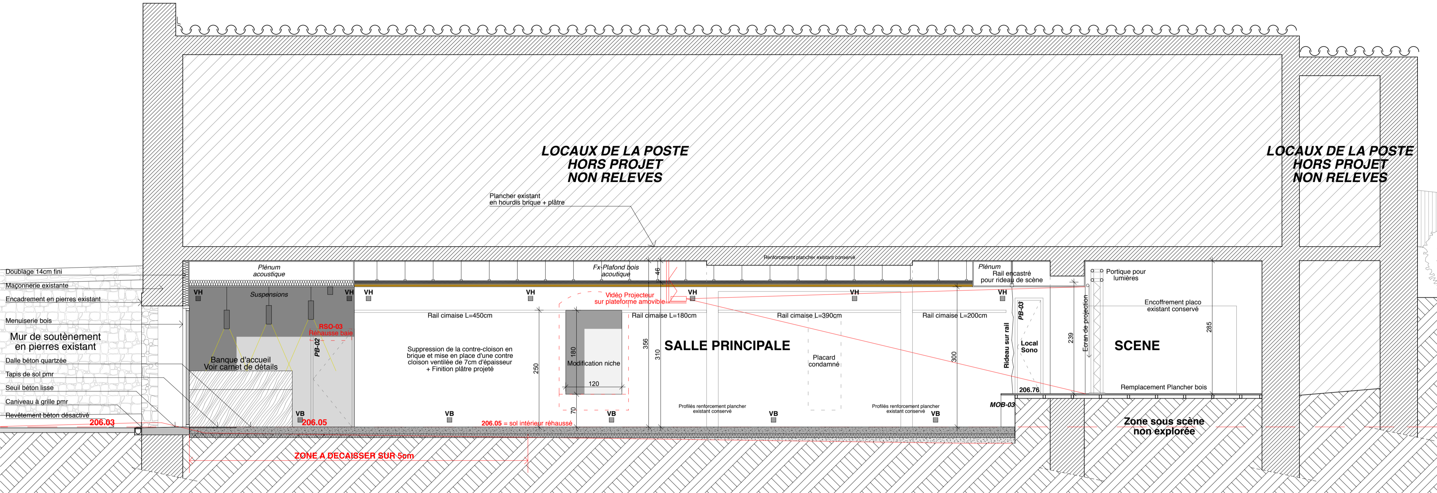
COUPE AA'
