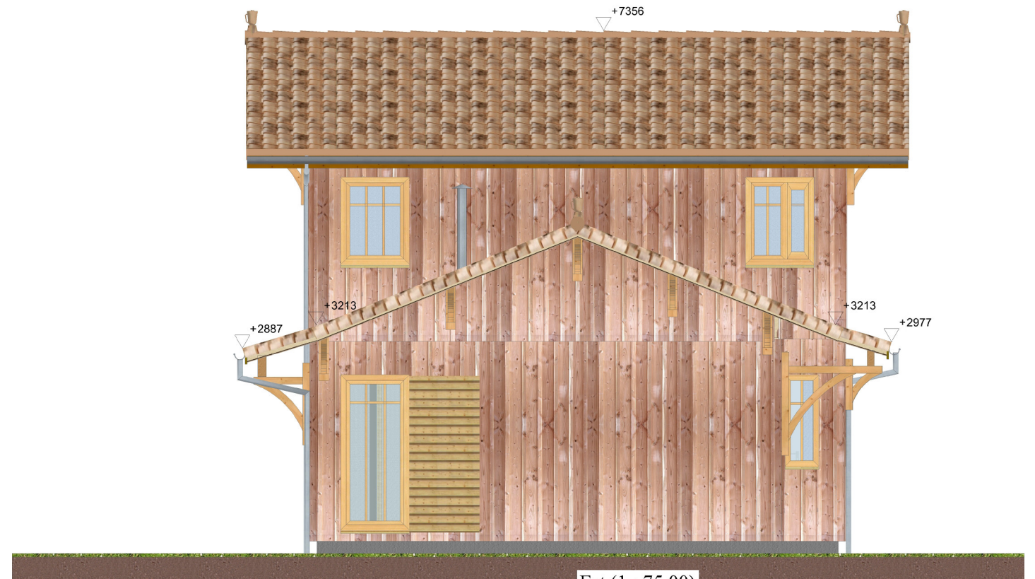
Est (1 : 75.00)
