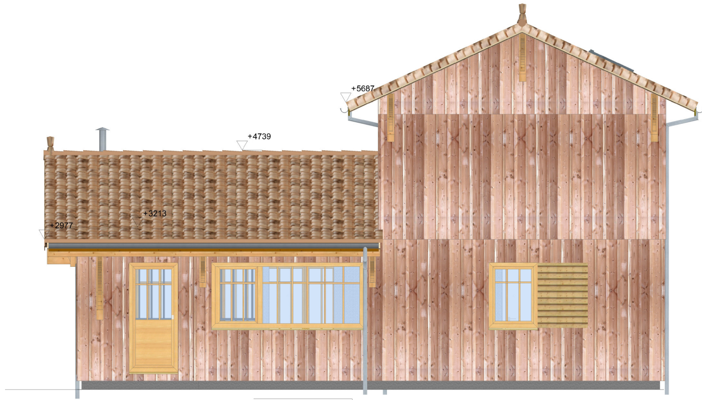
Nord (1 : 75.00)
