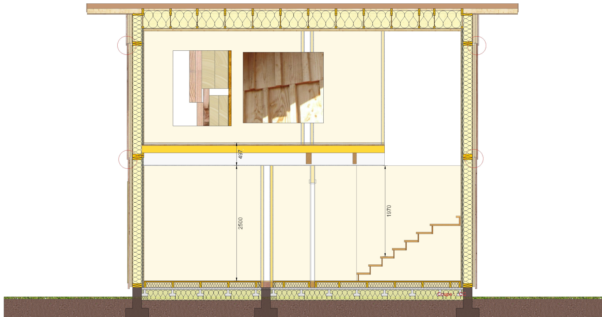
Coupe : CC (1 : 50.00)
