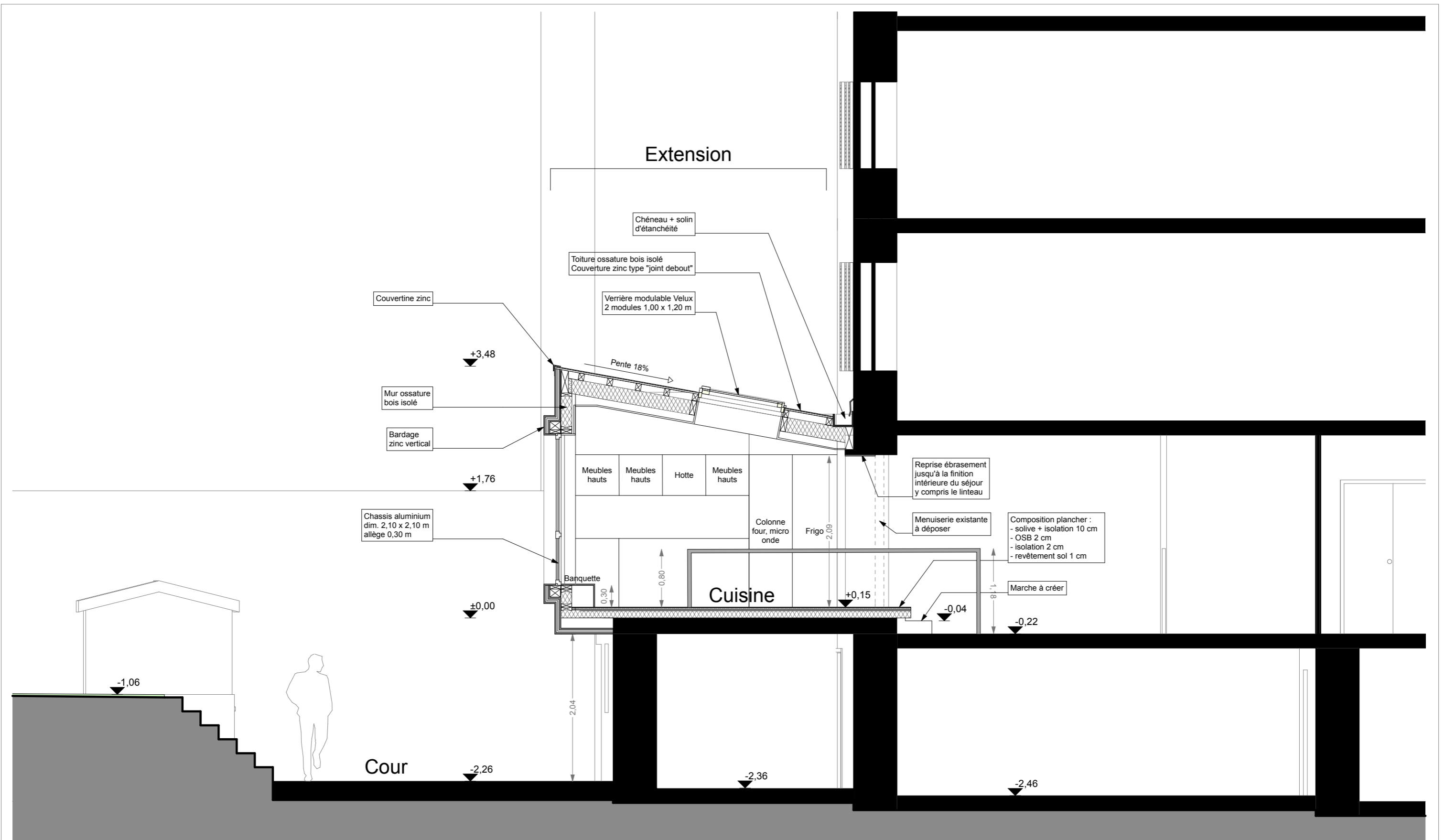
COUPE AA - état projeté
