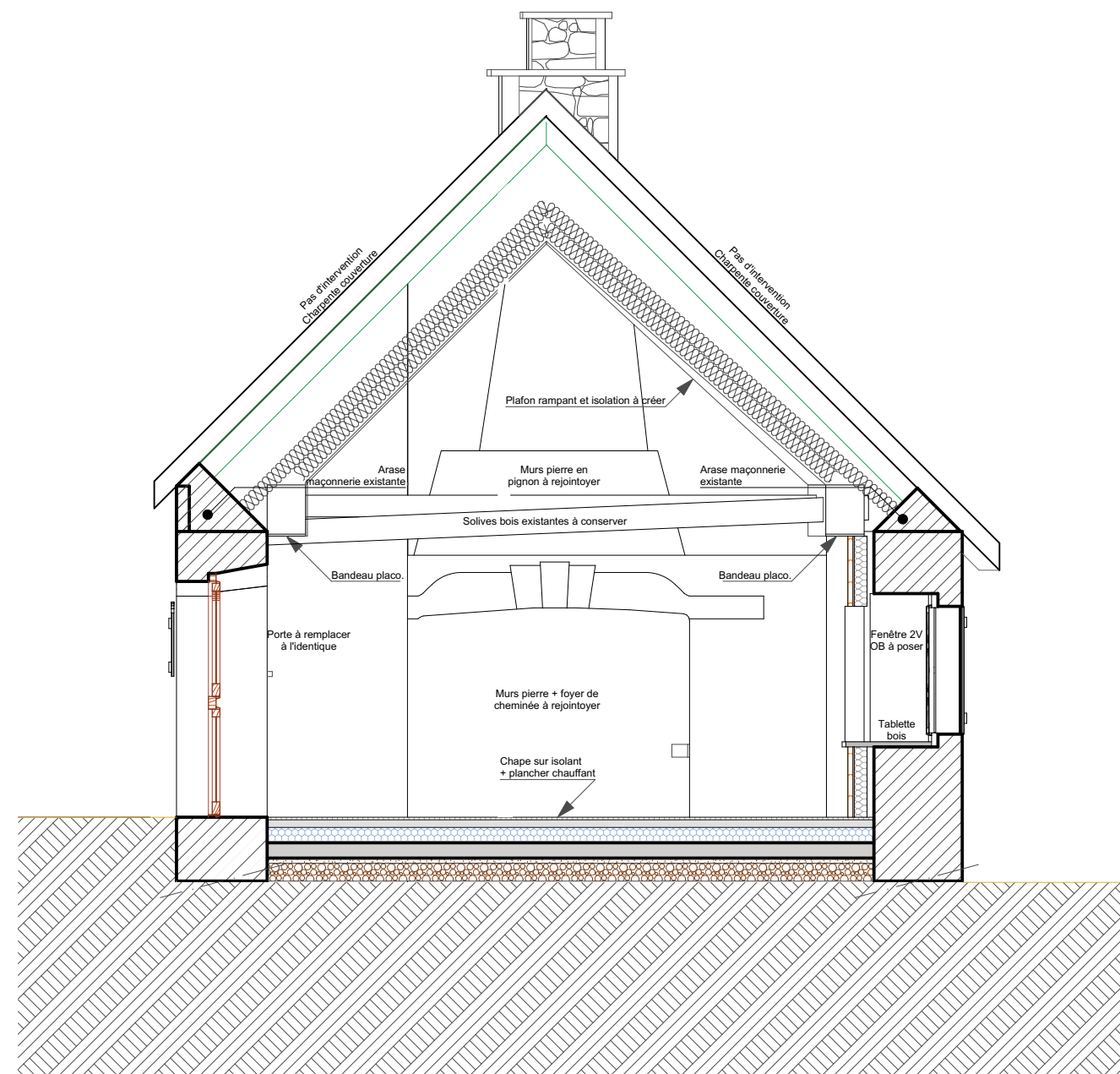
Coupe CC
