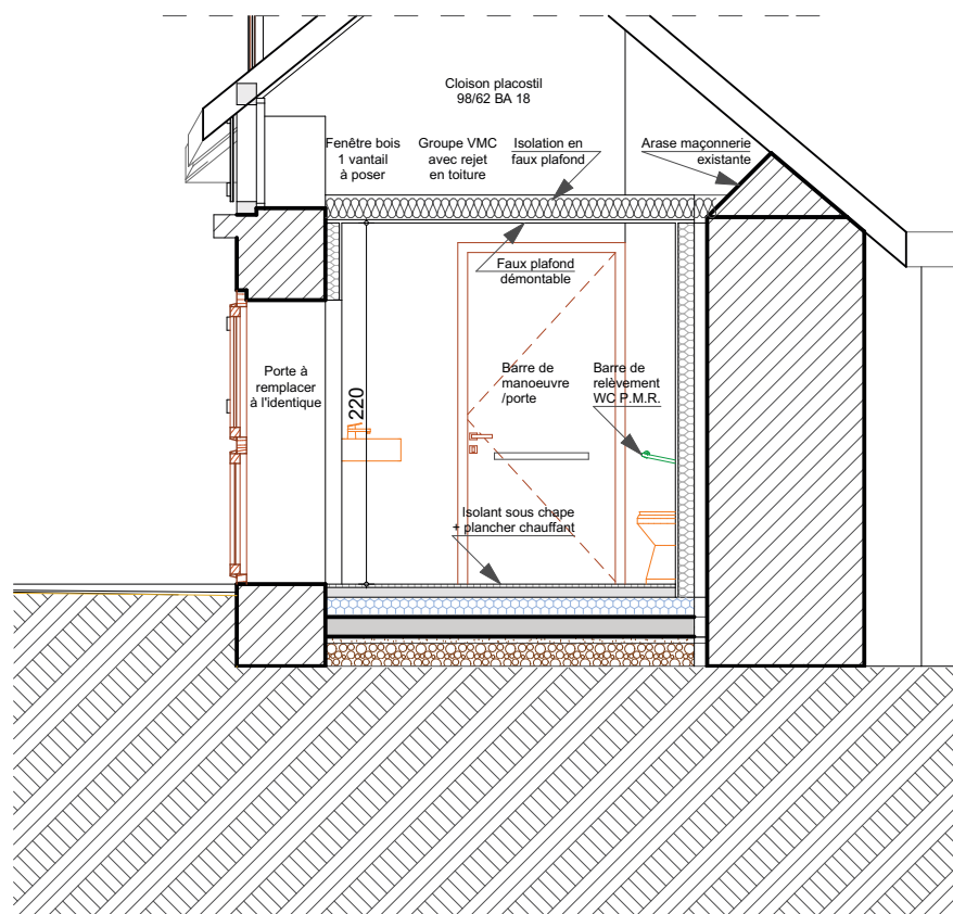
Coupe AA
