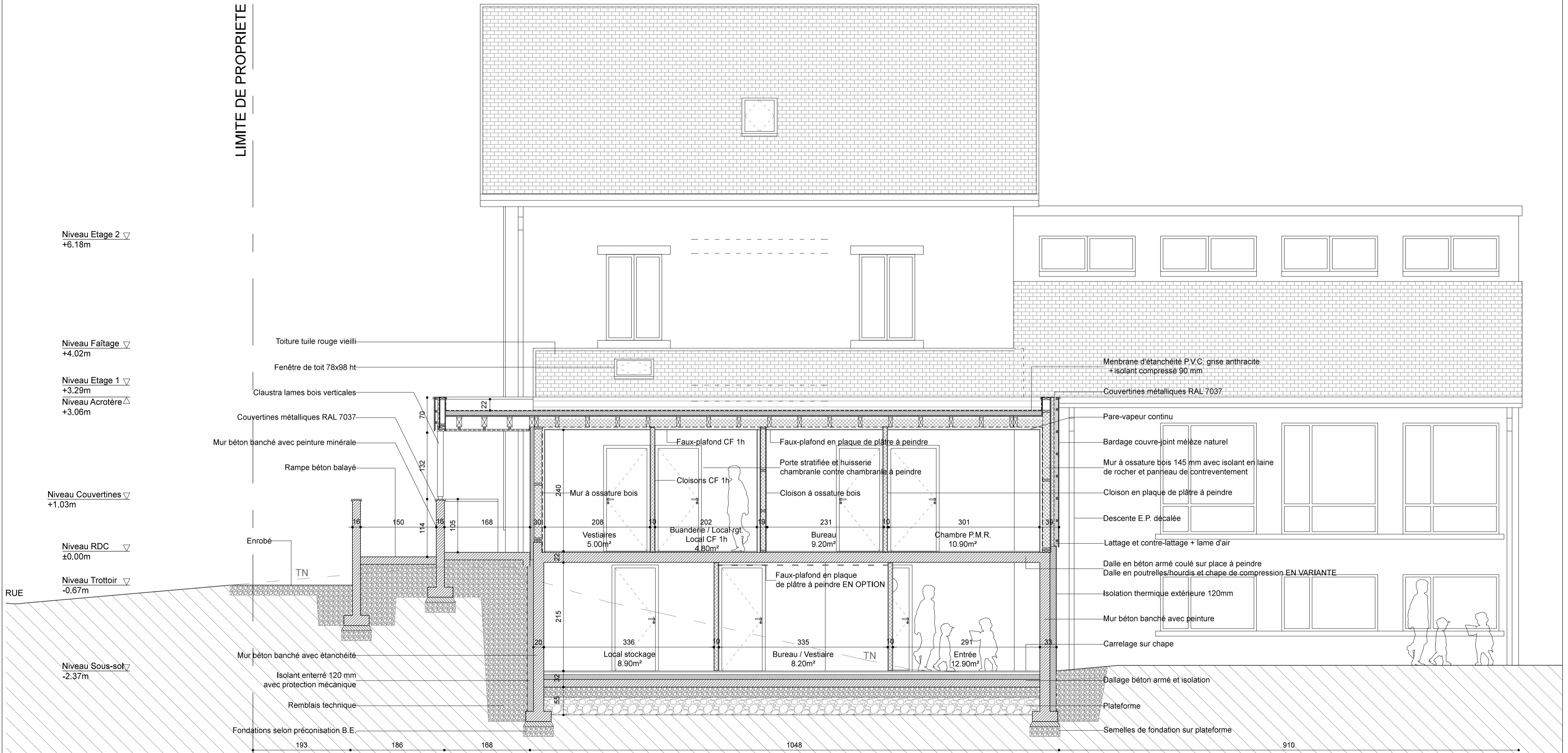
COUPE LONGITUDINALE
