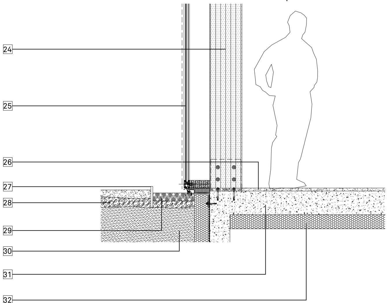
3. Détail coupe du rez-de-Chaussée
