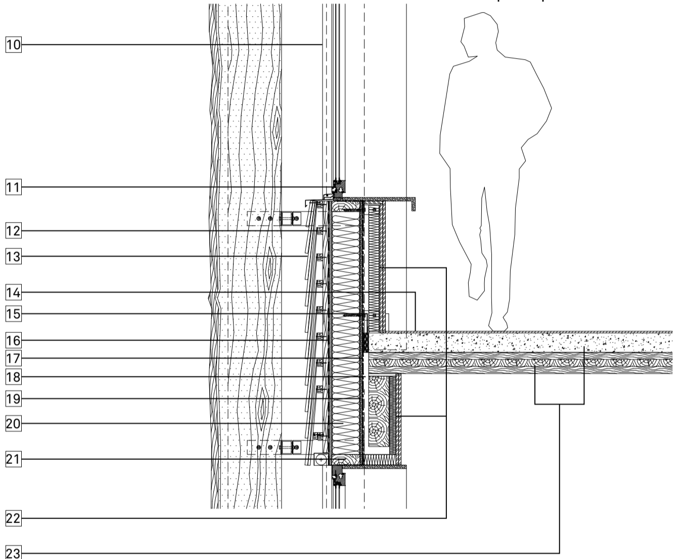
3. Détail coupe du rez-de-Chaussée
