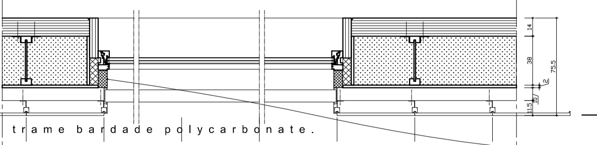
coupe horiz. AA
