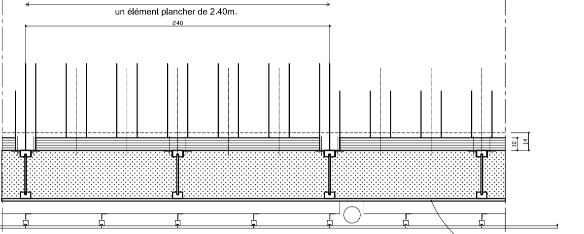
coupe horiz. CC
