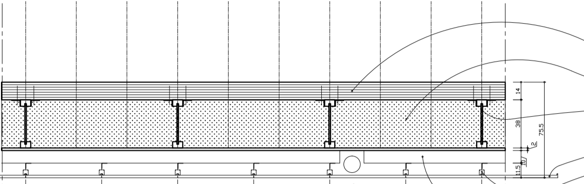
coupe horiz. BB
