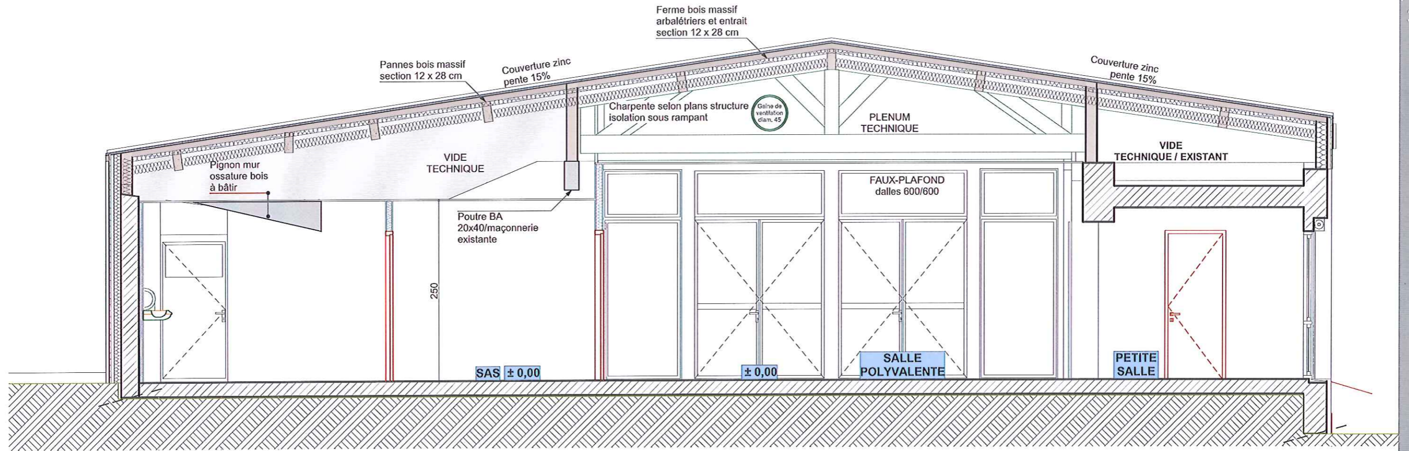
Coupe AA
