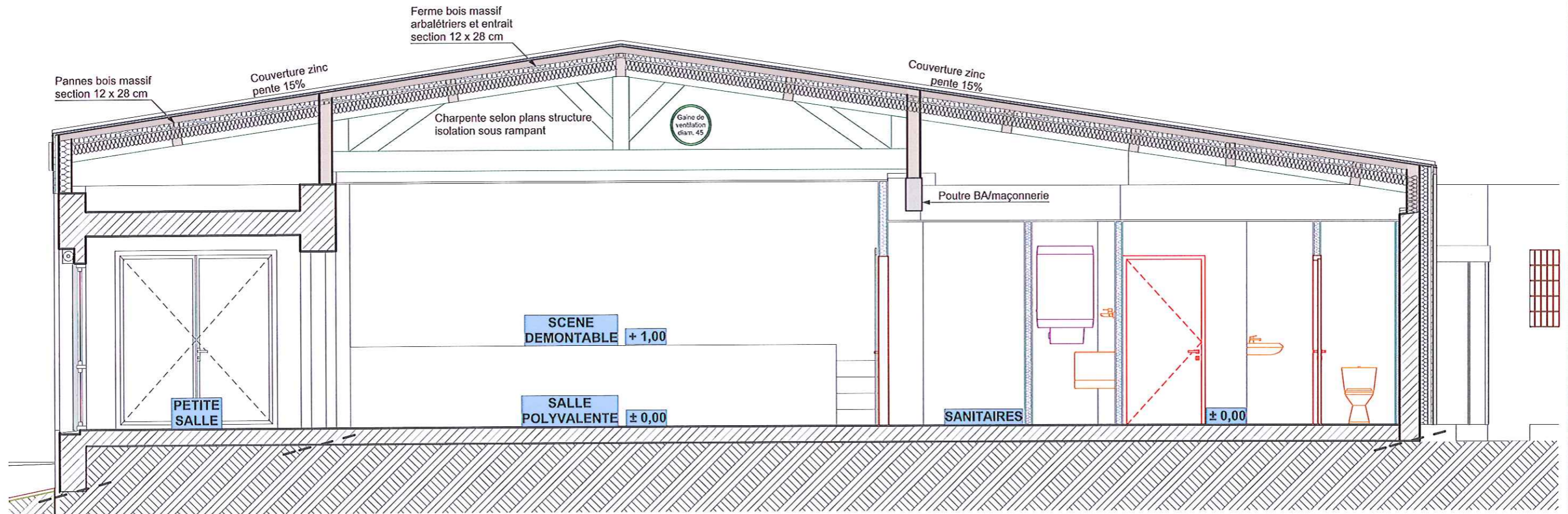
Coupe FF
