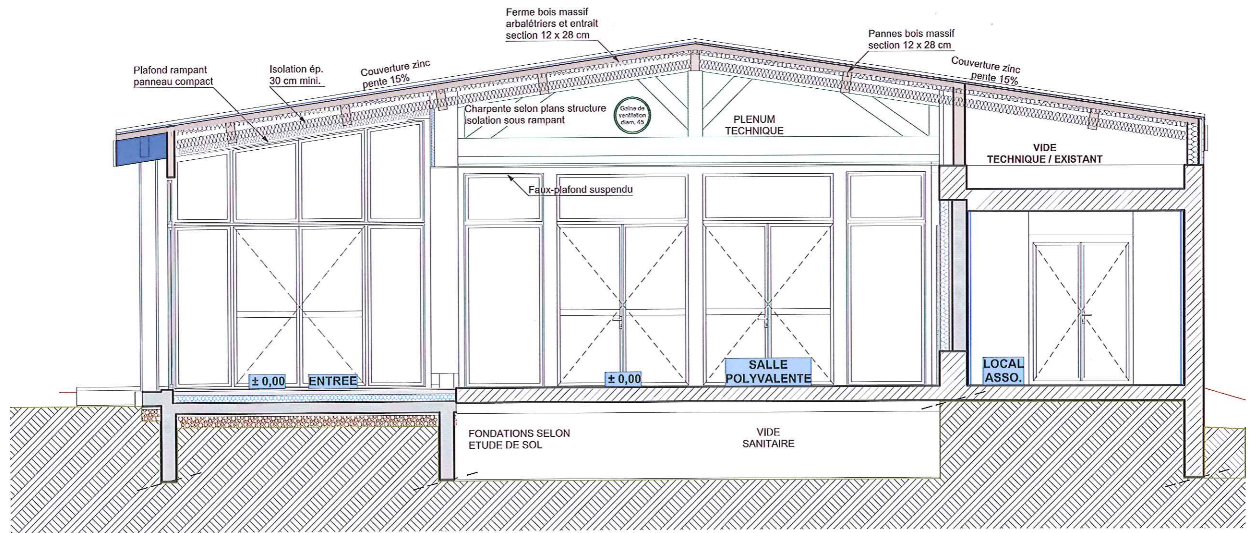
Coupe CC
