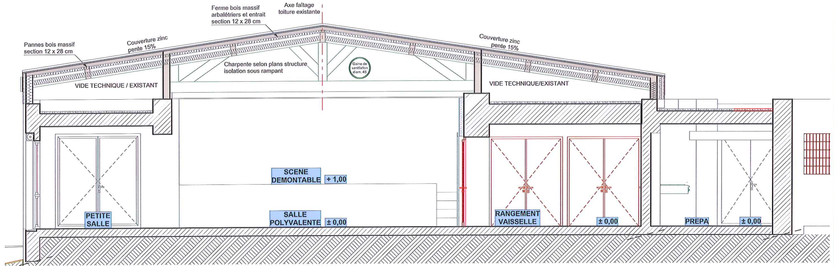
Coupe BB
