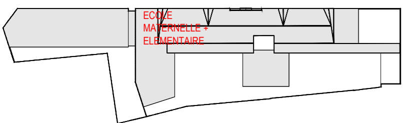
Plan du RDC ECOLE MATERNELLE ET ELEMENTAIRE _ Ech : 1/200e
