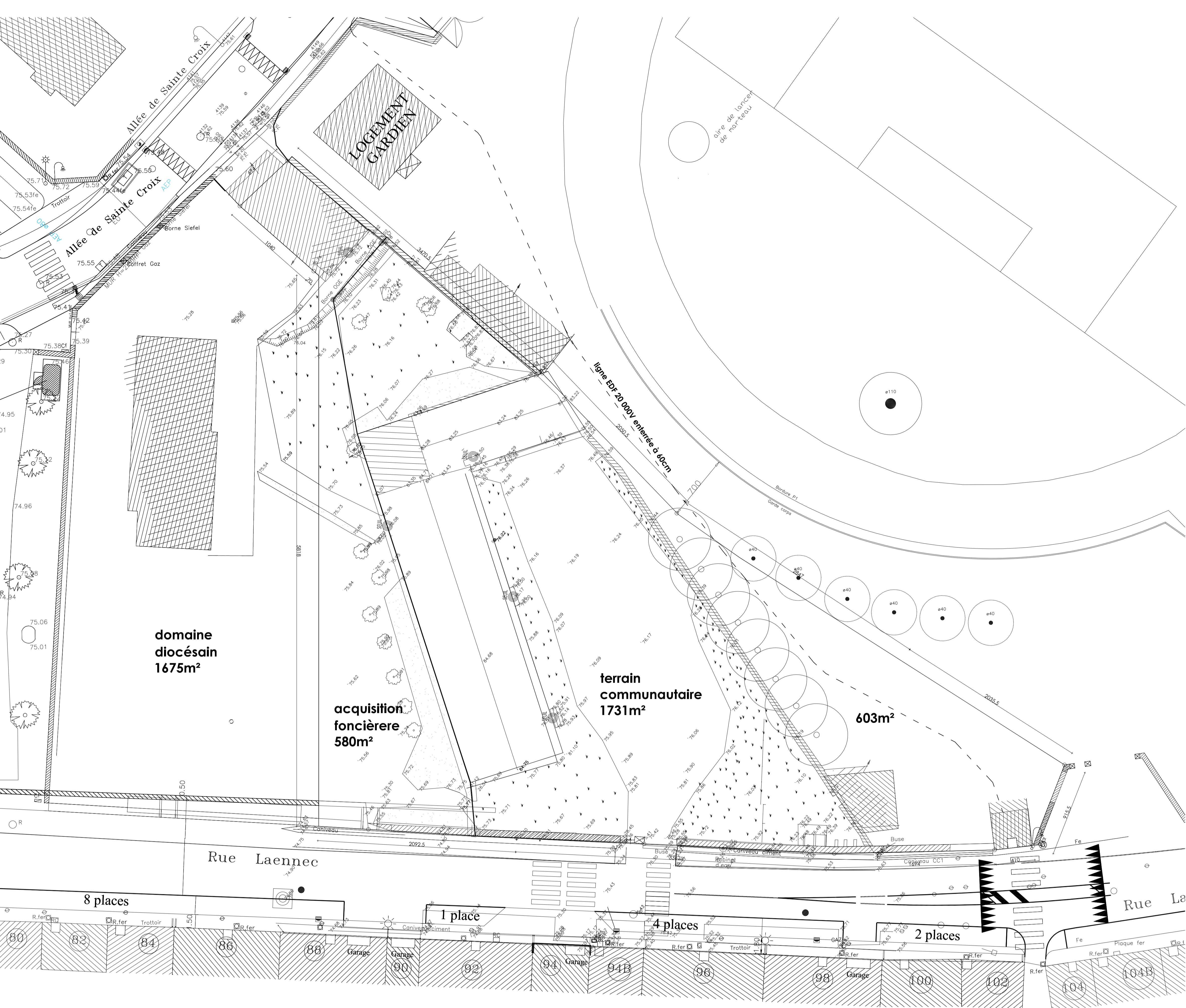
Vue en plan de masse existant 0 10 m 25 m
