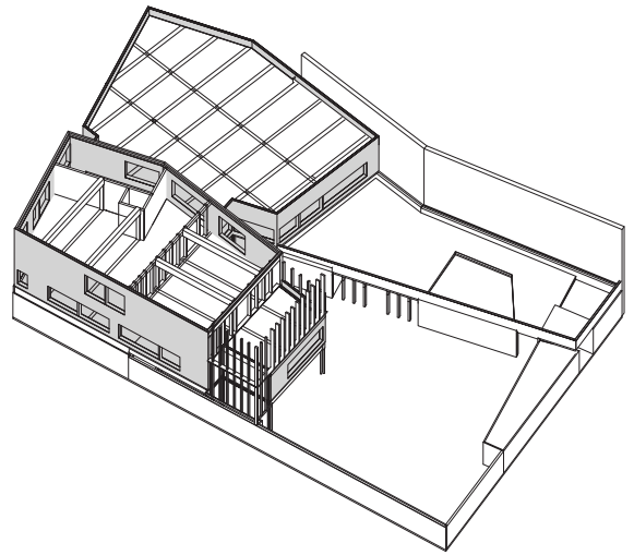
Murs à ossature bois & Isolation Paille et Laine de bois
