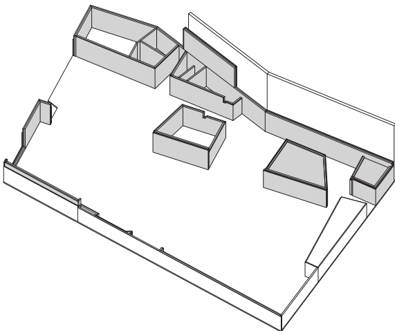
Voiles en Béton armé
