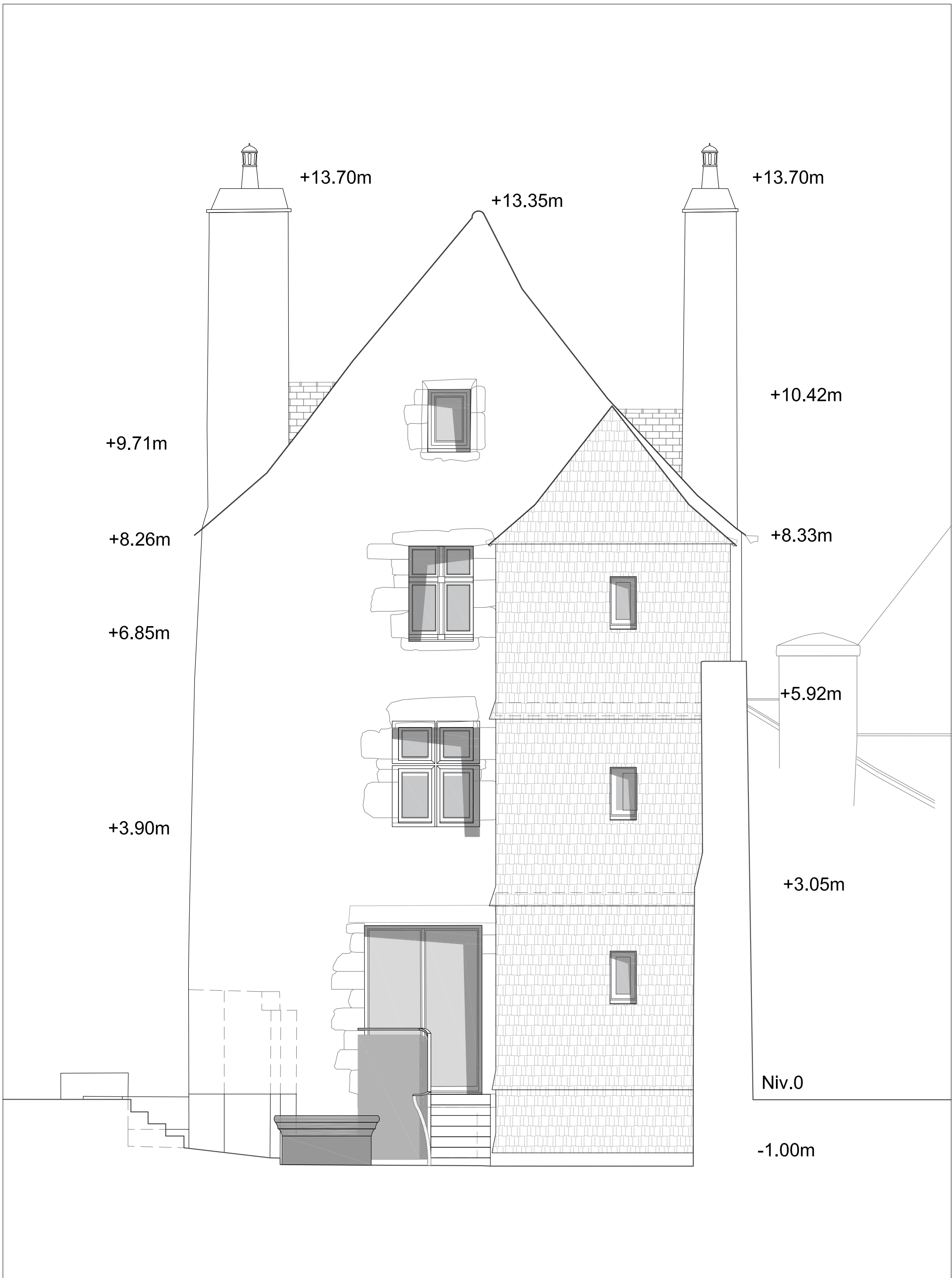
PROJET : Façade Nord - Echelle : 1/50e
