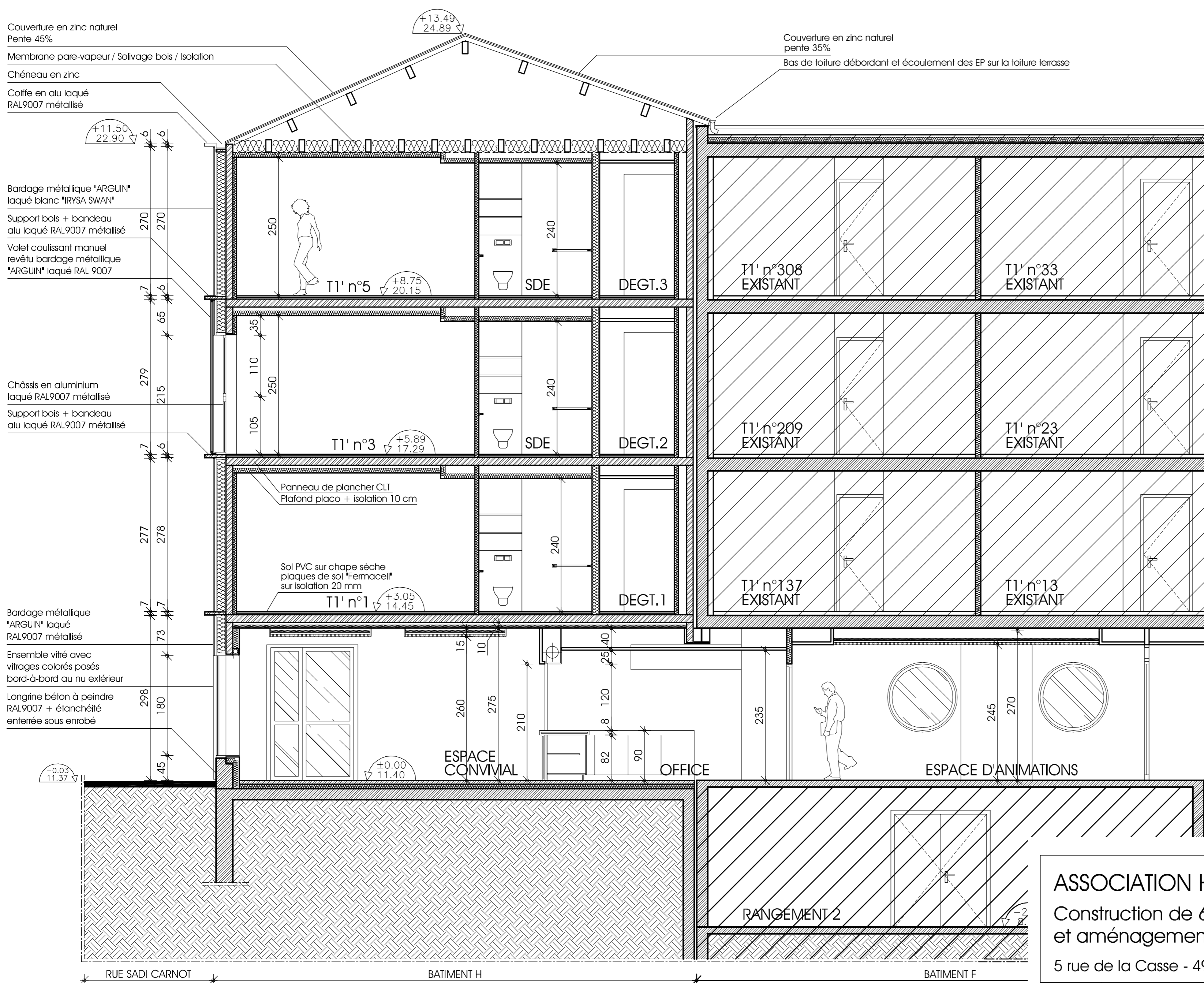
COUPE C2 - 1/50
