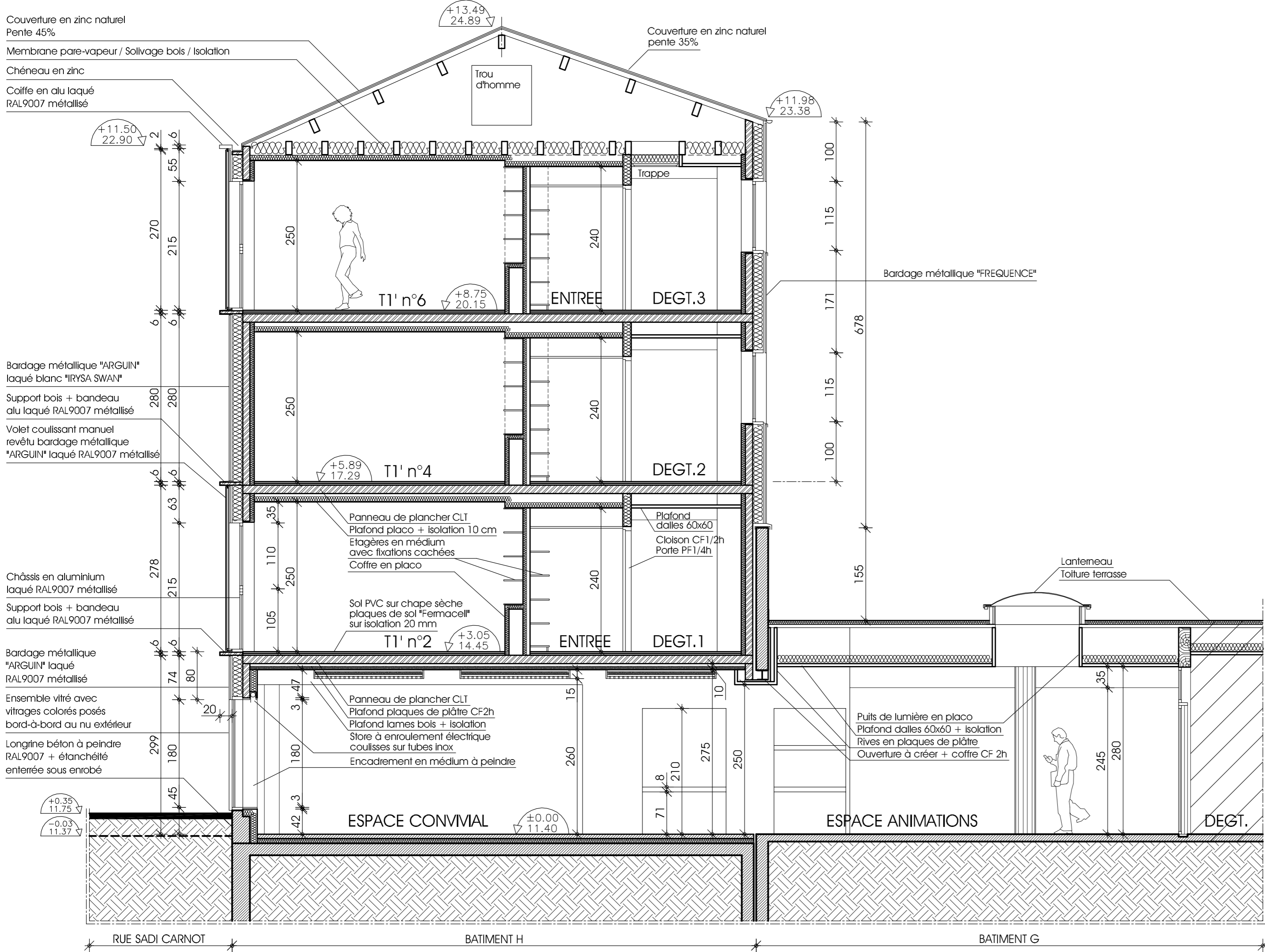
COUPE C1 - 1/50
