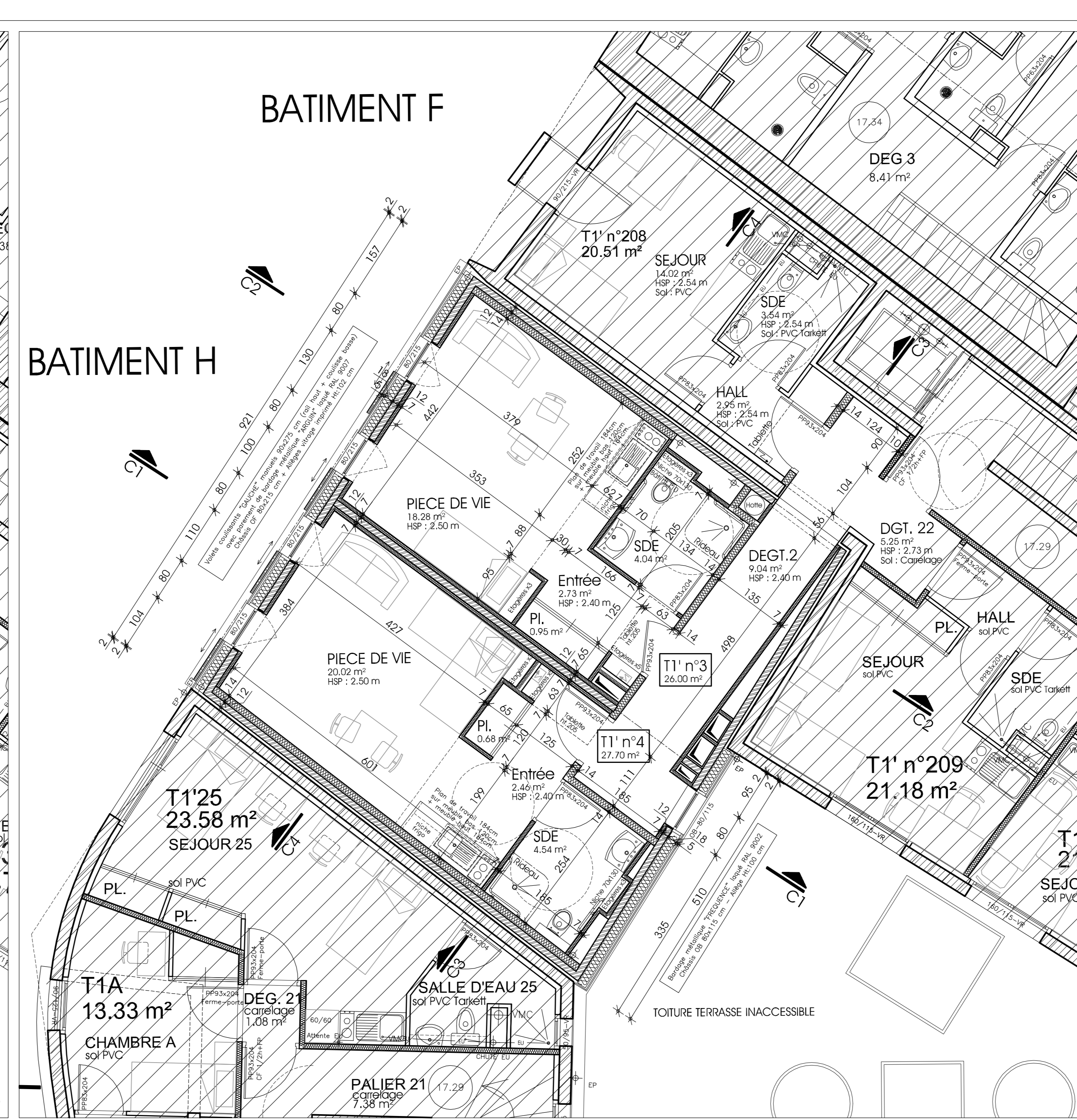
PLAN ETAGE 2 - 1/50
