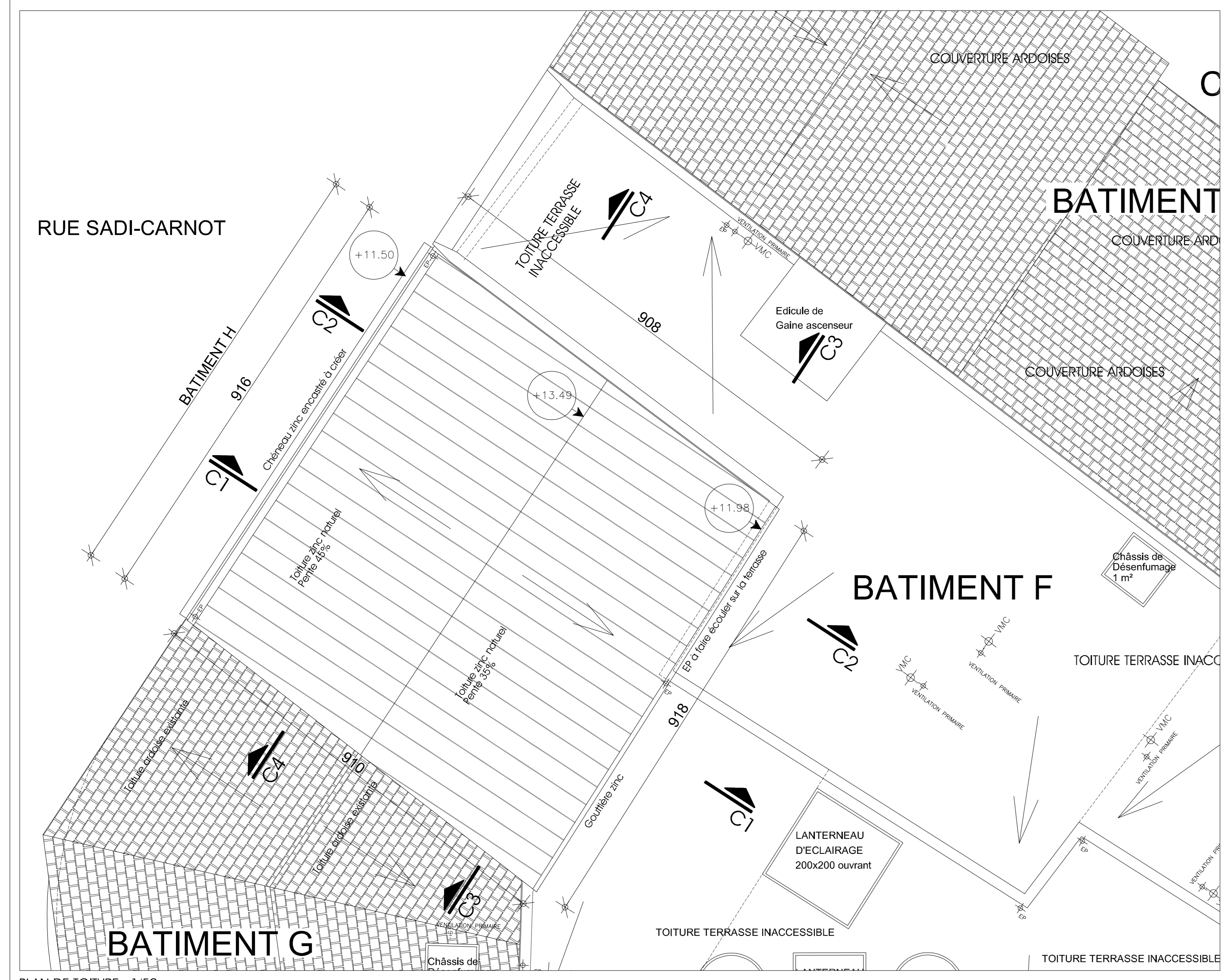
PLAN DE TOITURE - 1/50
