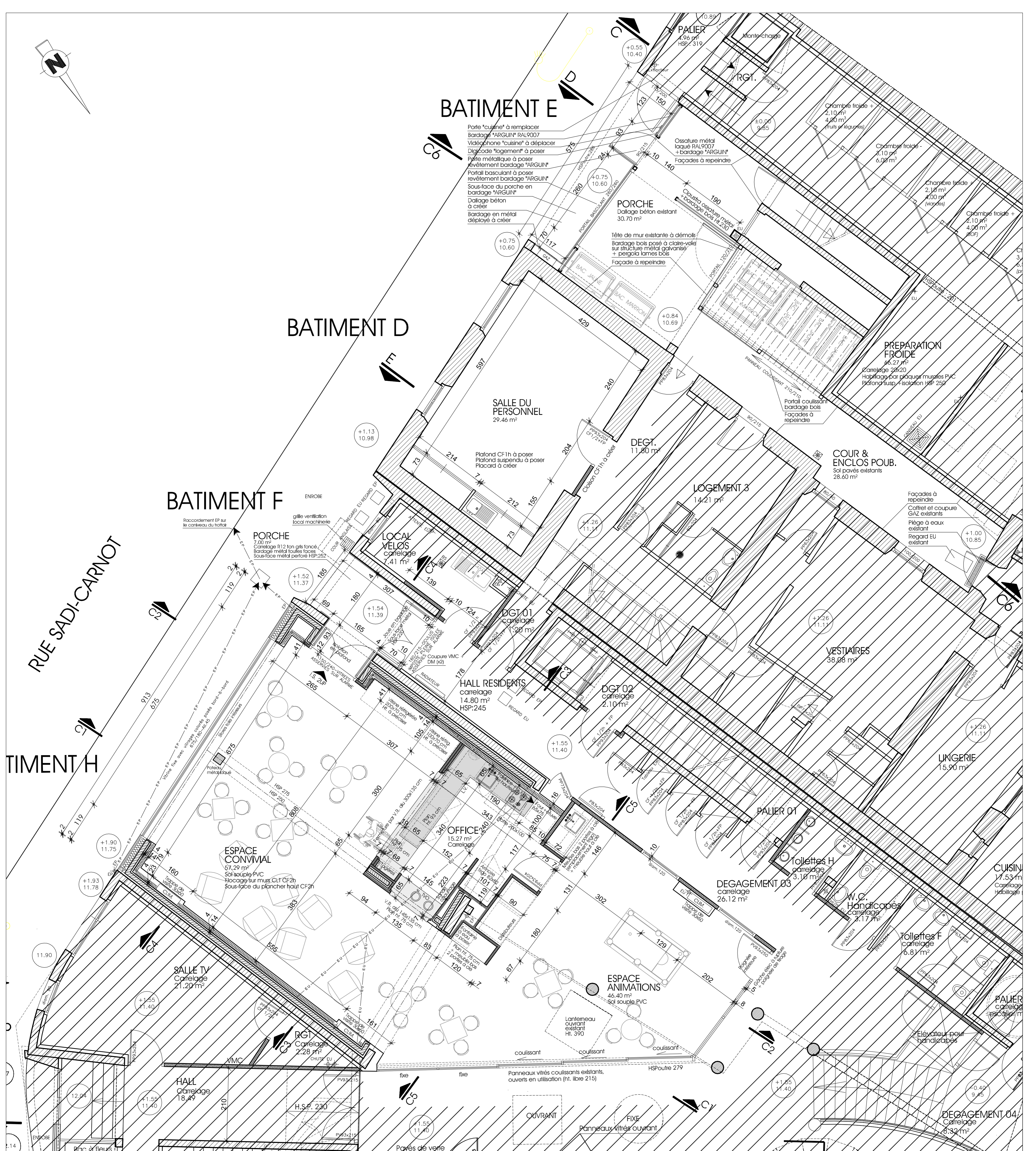
PLAN REZ-DE-CHAUSSEE - 1/50
