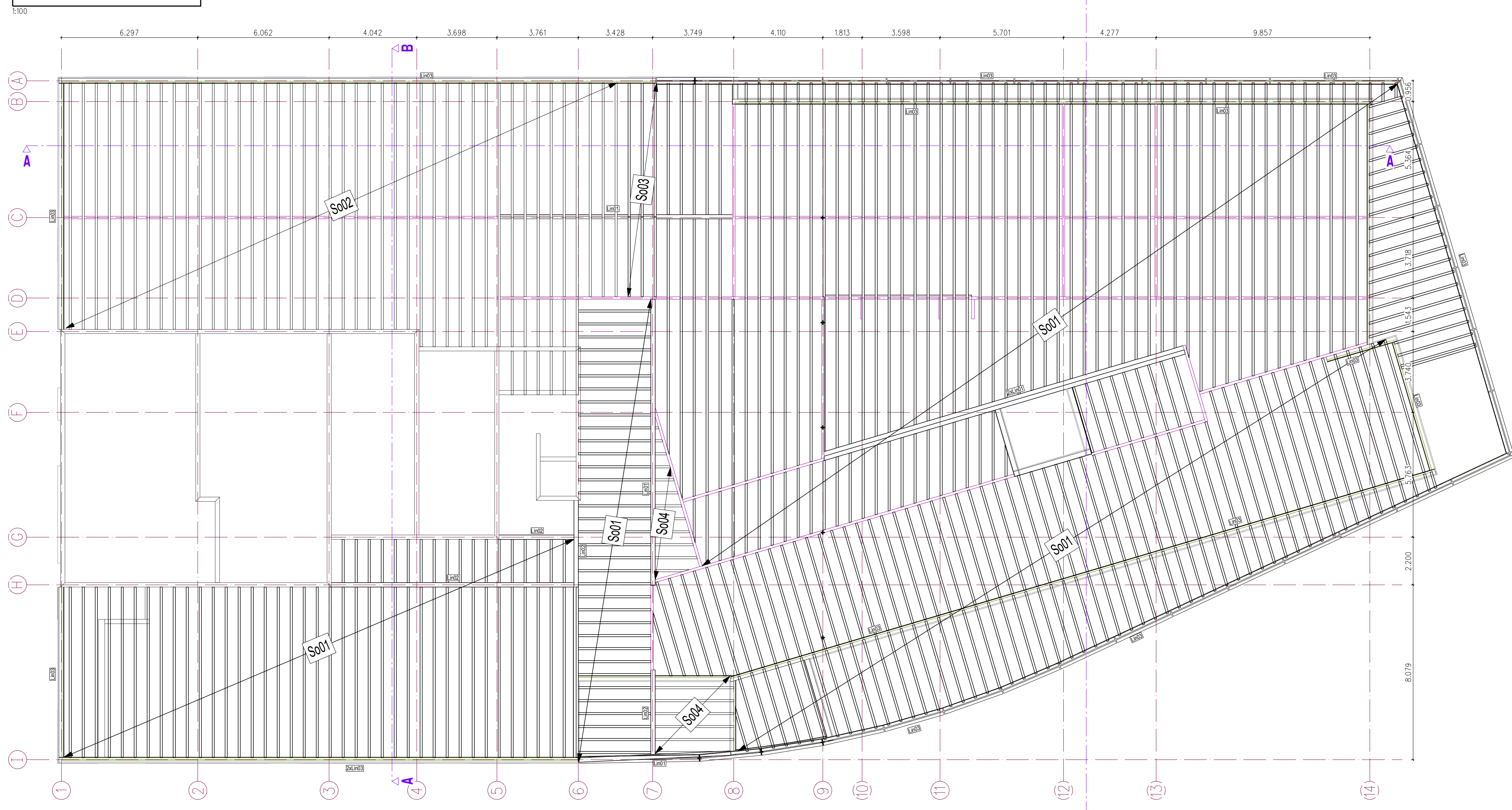
Plan de Plancher
