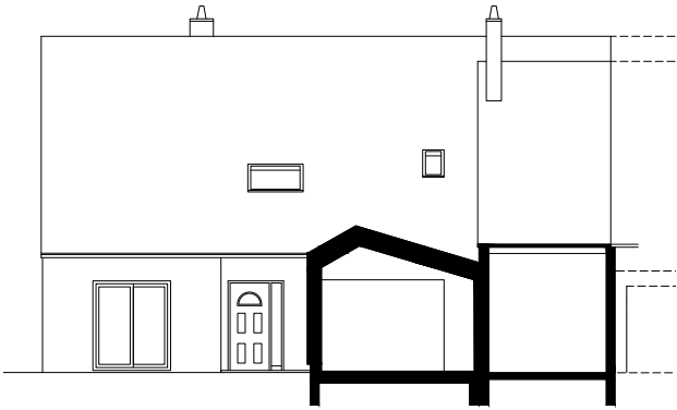
COUPE TRANSVERSALE
