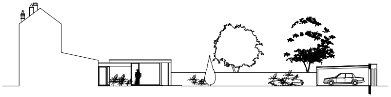
COUPE TRANSVERSALE
