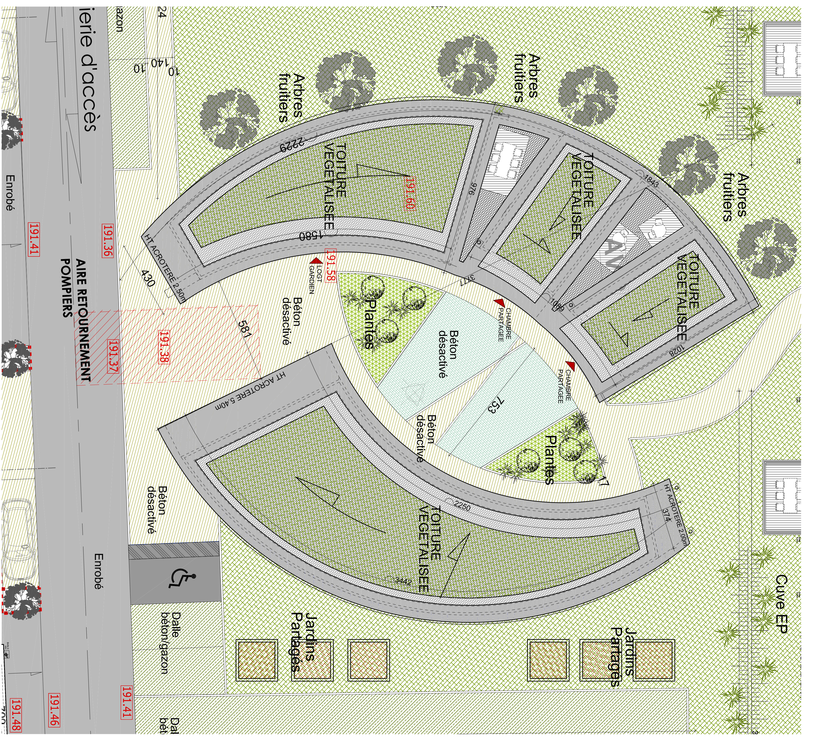
PLAN TOITURE 1/100ème
