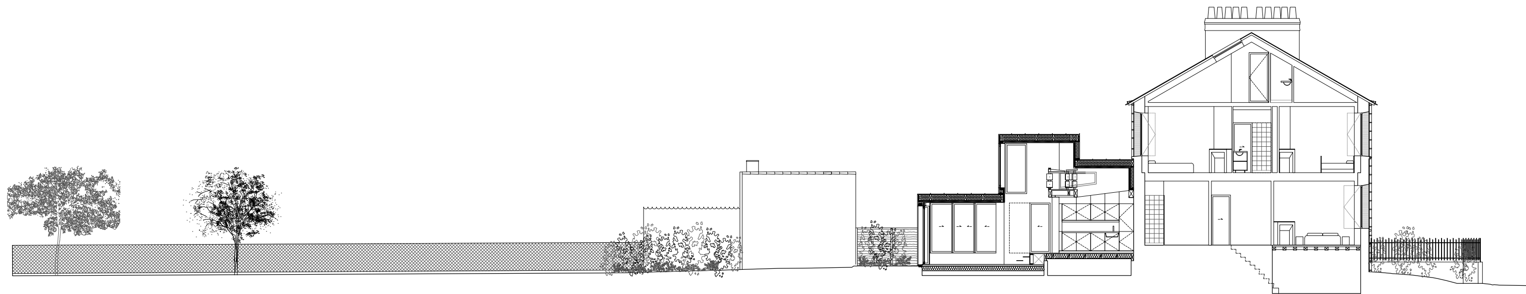
COUPE F 0 1.5 3 6
