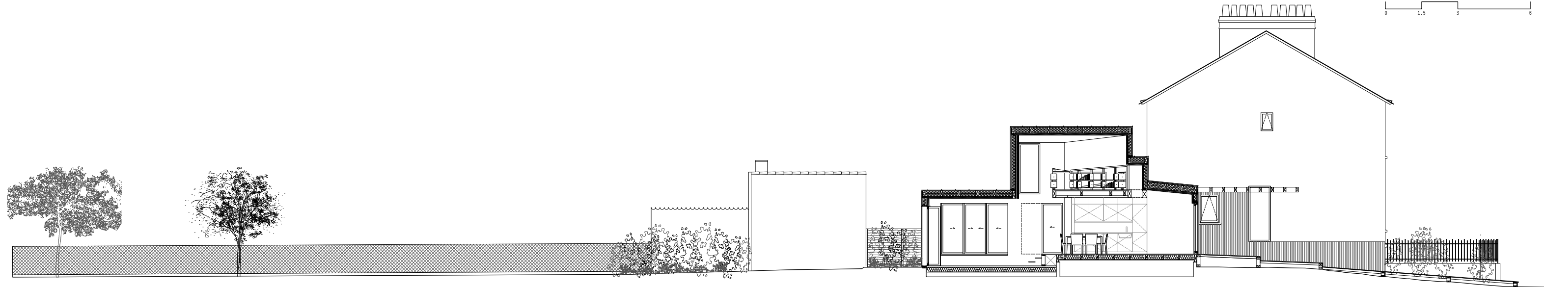
COUPE G 0 1.5 3 6
