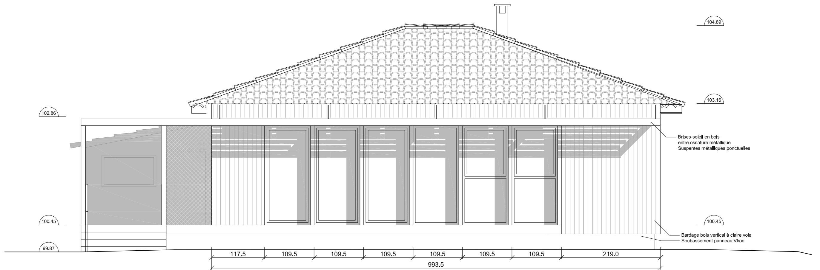
ELEVATION SUD
