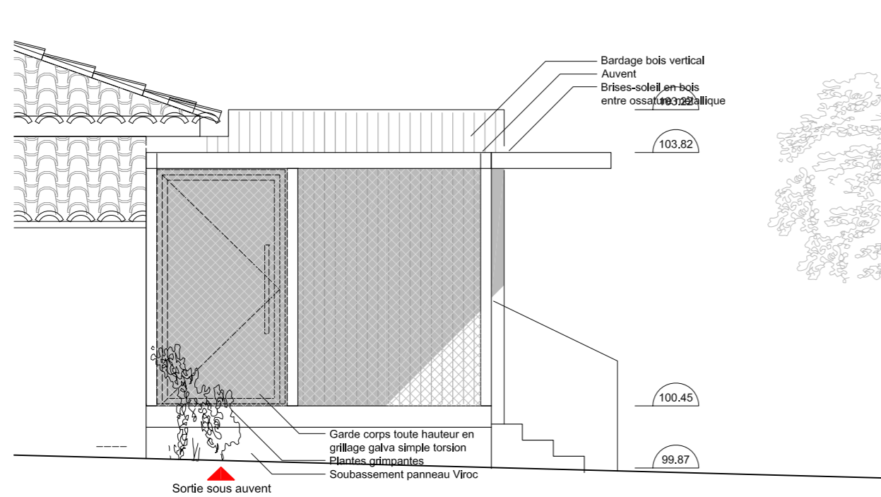
ELEVATION OUEST
