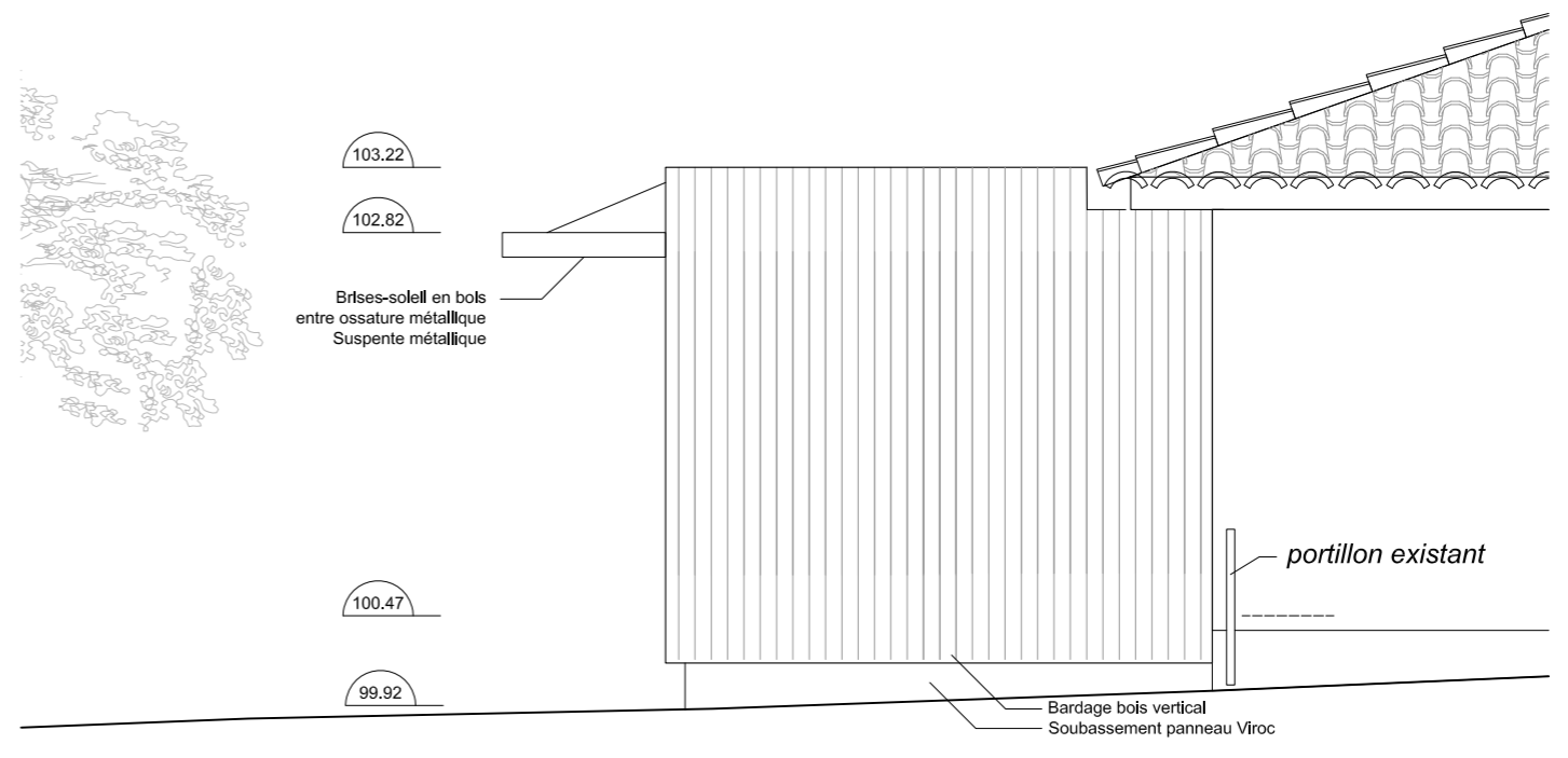
ELEVATION EST
