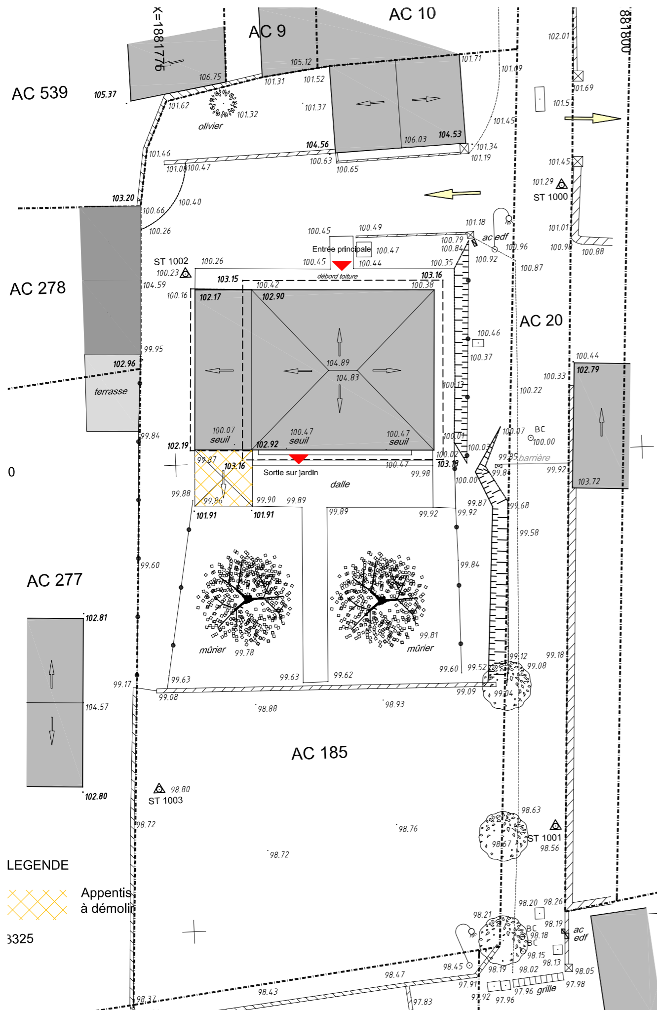
PLAN MASSE ETAT DES LIEUX Extrait relevé topographique Cabinet PERNOT
