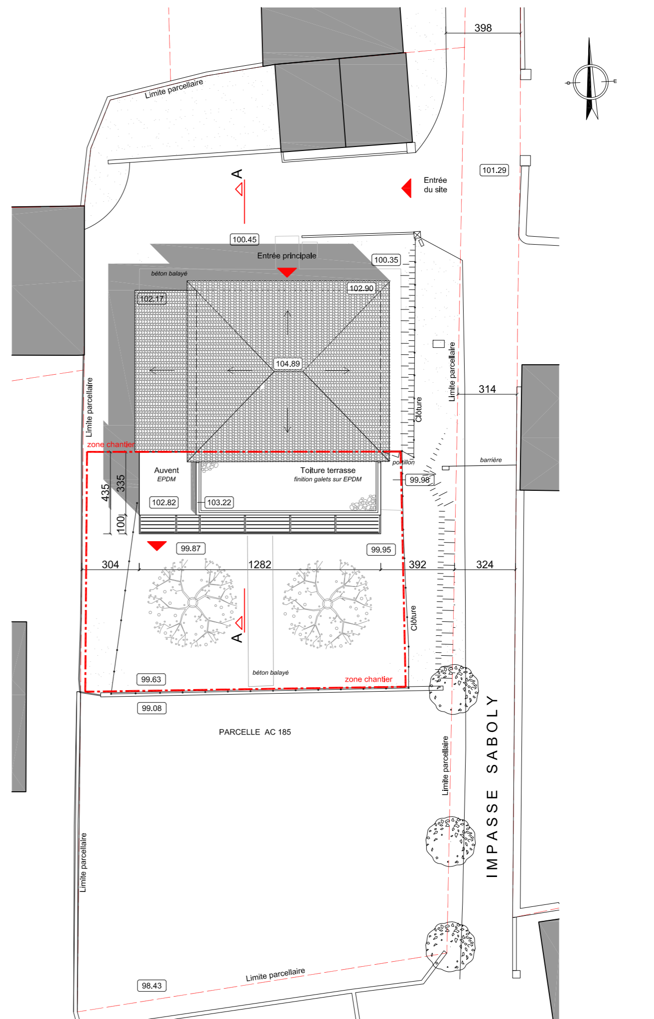
PLAN MASSE PROJET
