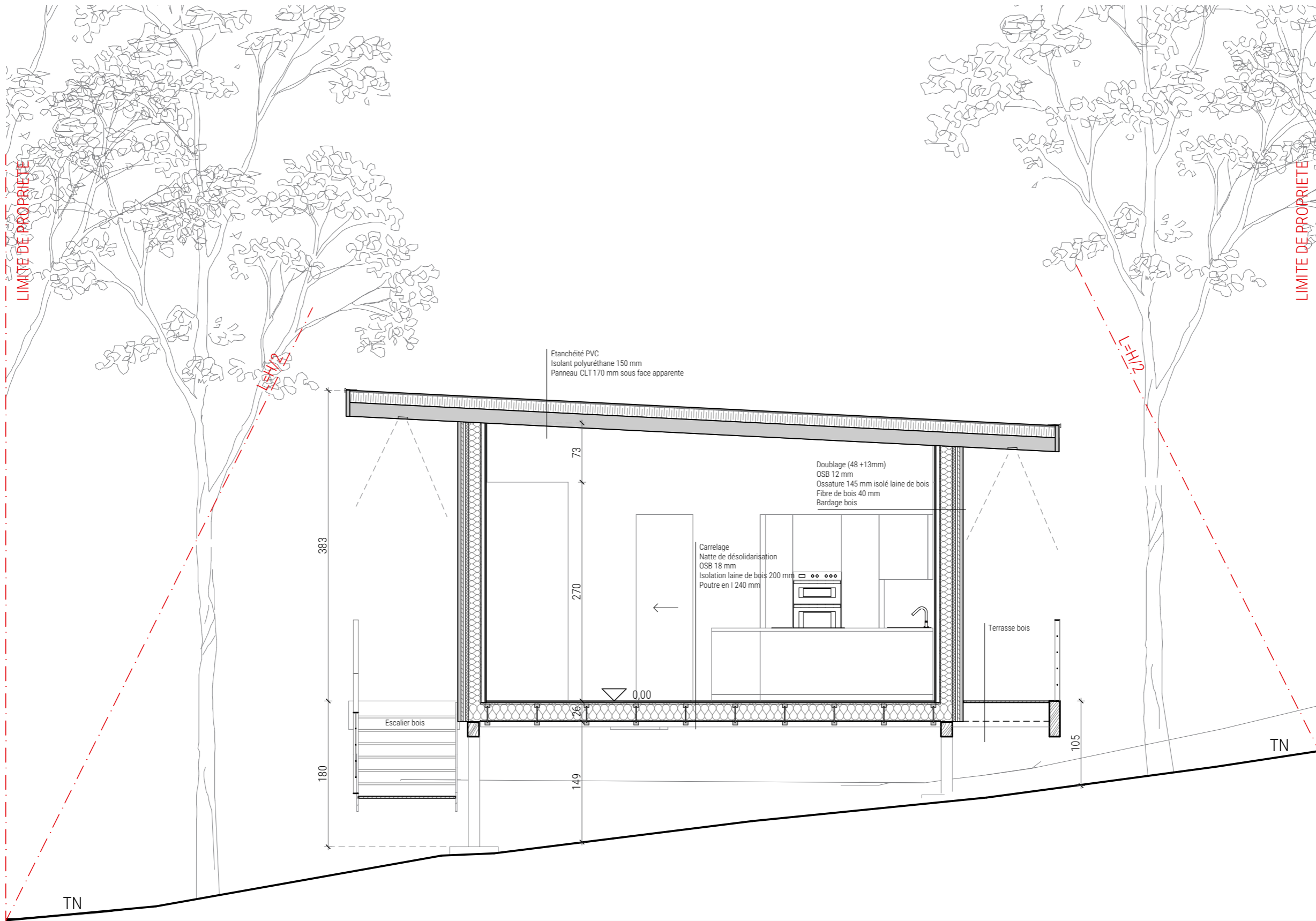
COUPE BB 1/50
