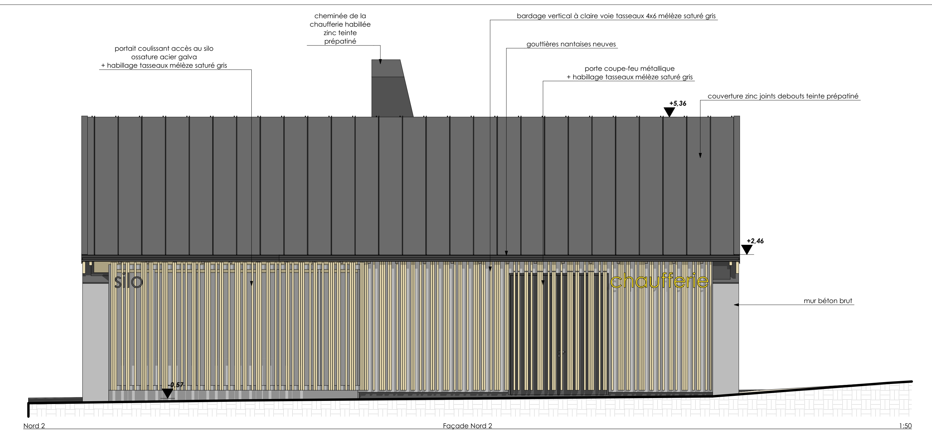
Nord 2 Façade Nord 2 1:50
