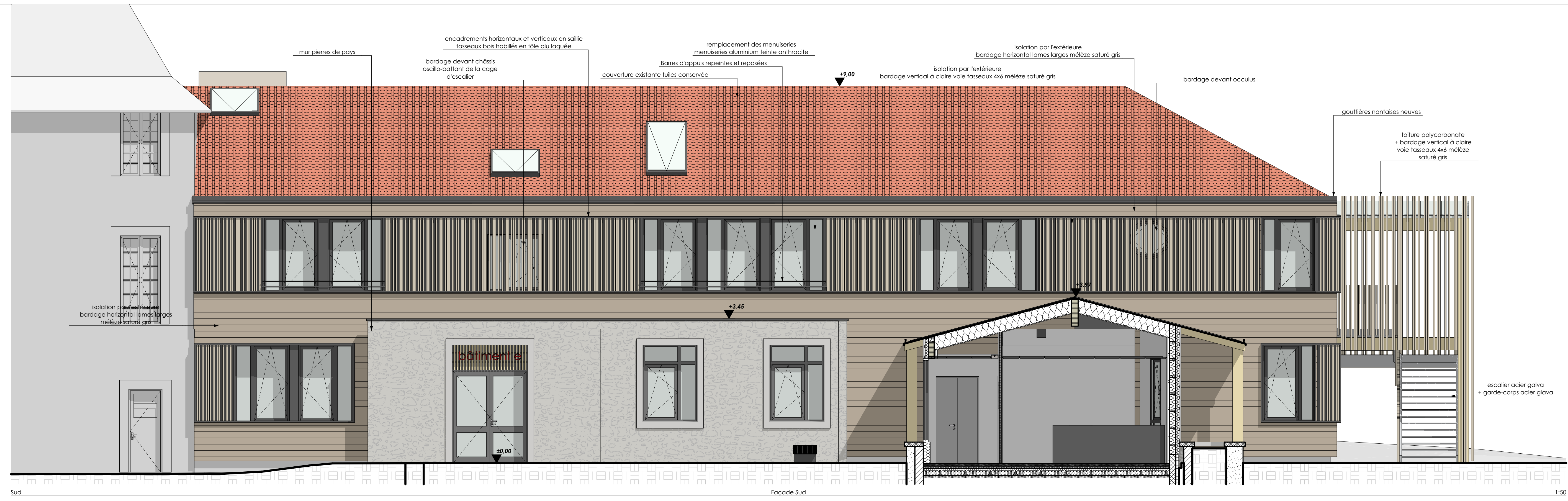
Sud Façade Sud 1:50
