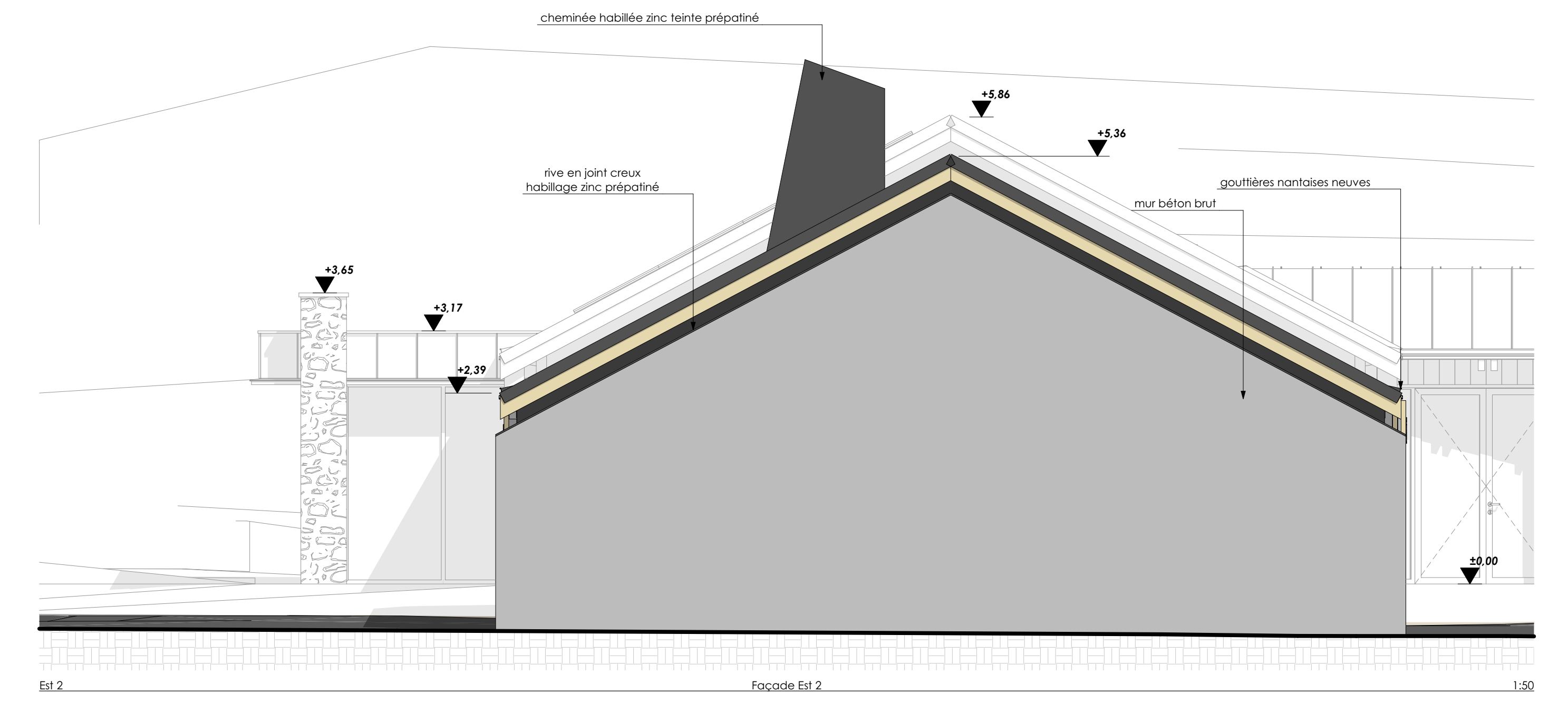
Est 2 Façade Est 2 1:50
