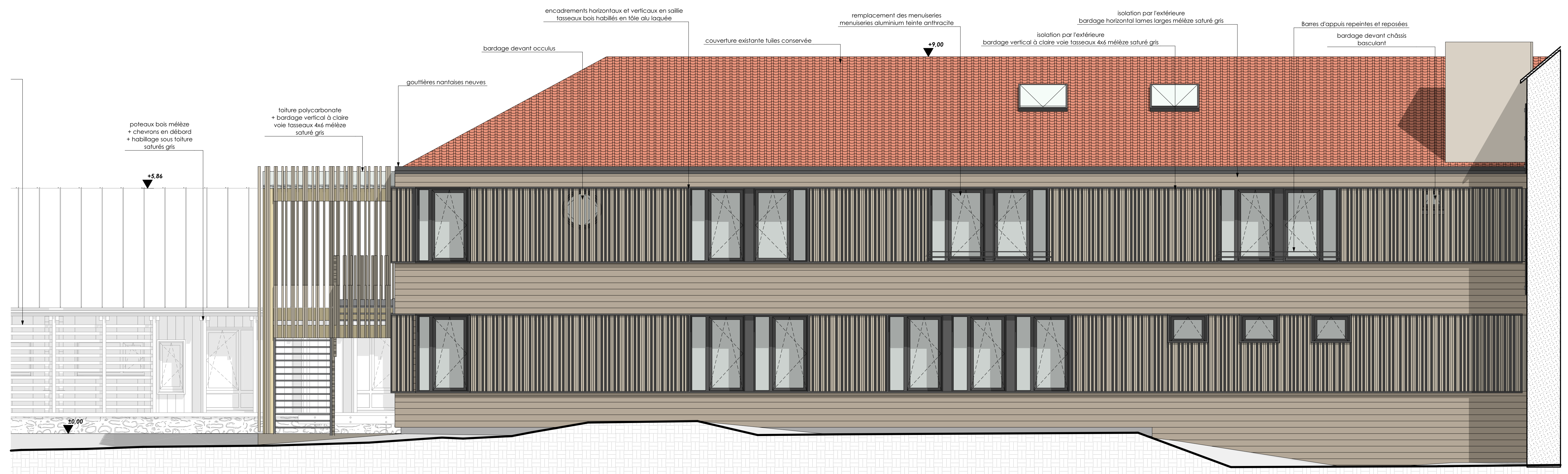
Nord Façade Nord 1:50
