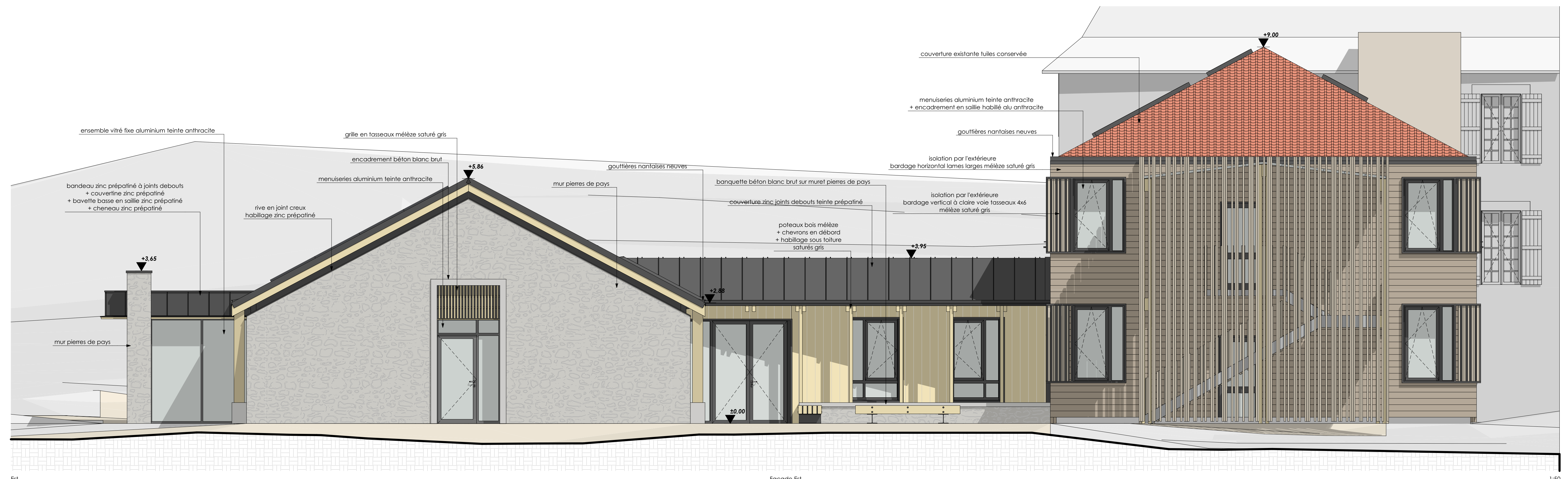
Est Façade Est 1:50
