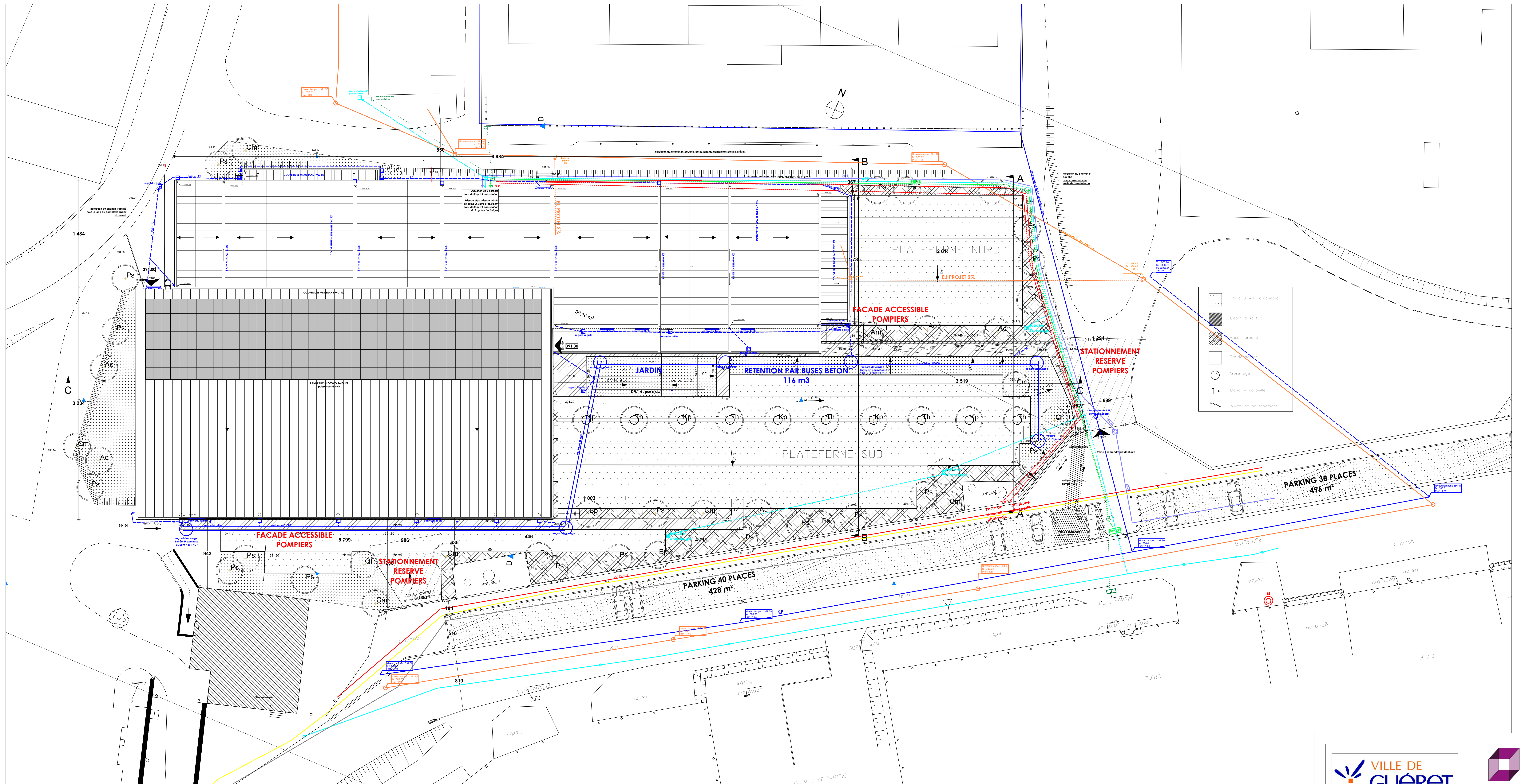
PLAN DE MASSE - PLAN DES RESEAUX 1/200
