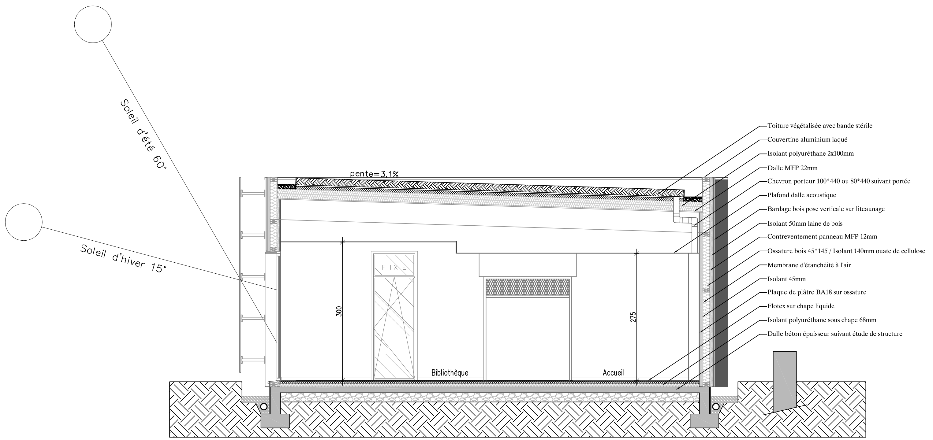
Coupe HH
