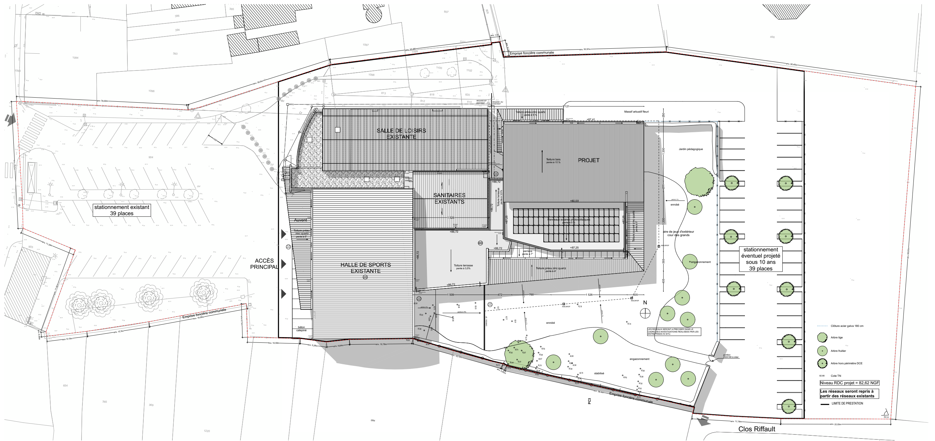
PLAN DE MASSE PROJET 1/200e
