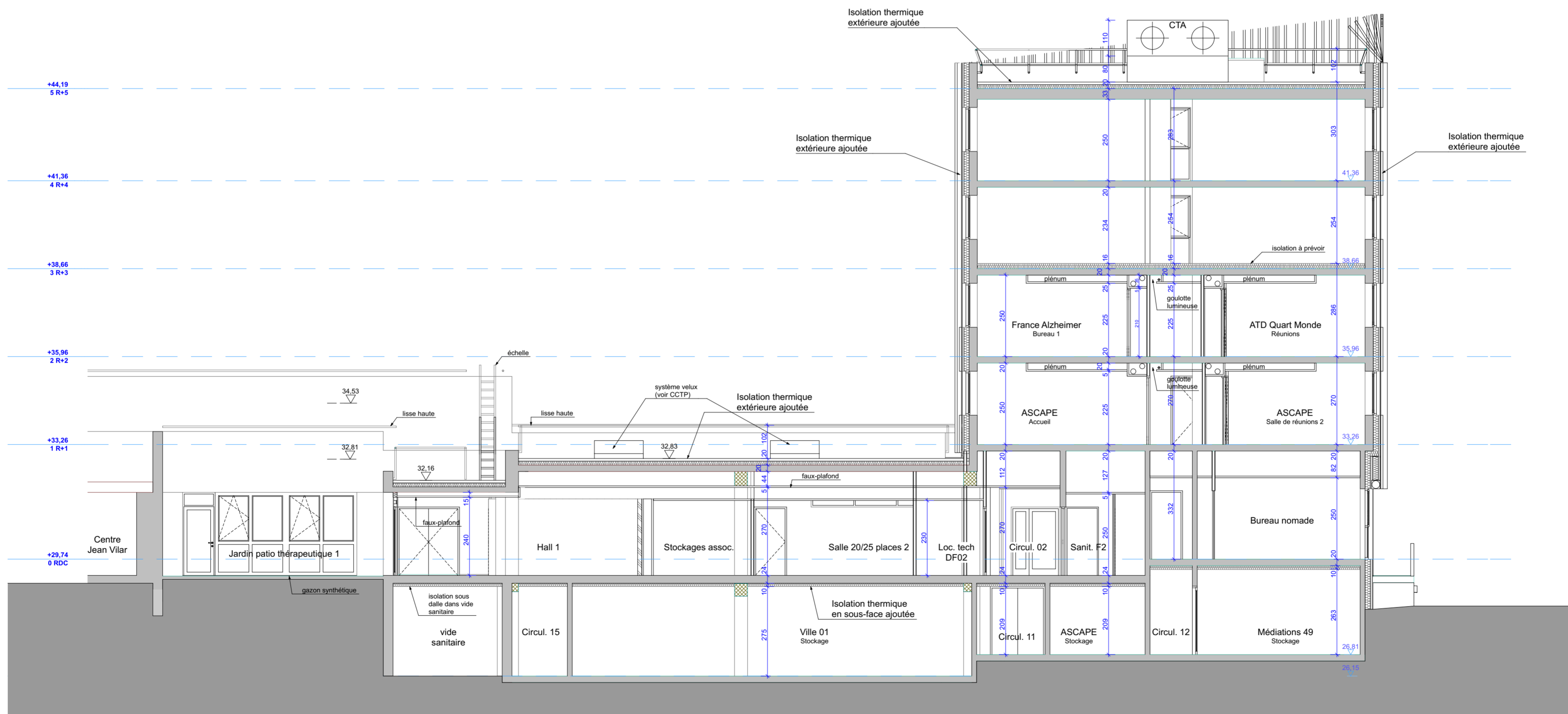
Coupe AA
