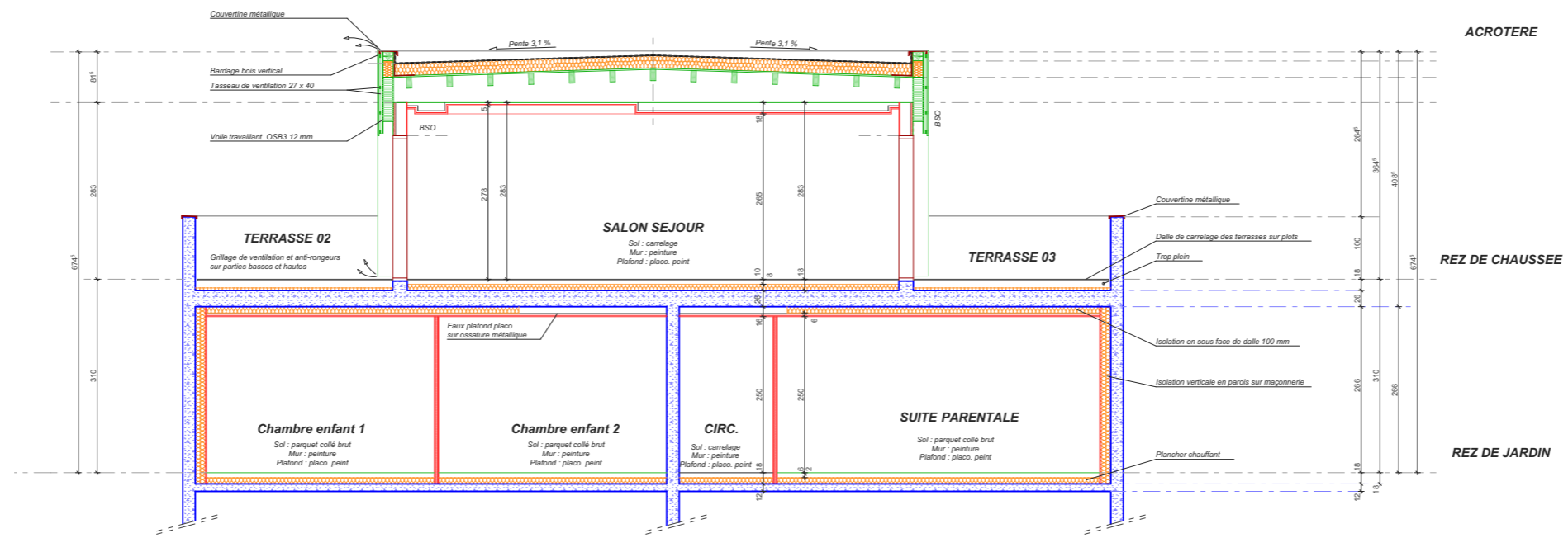
COUPE AA
