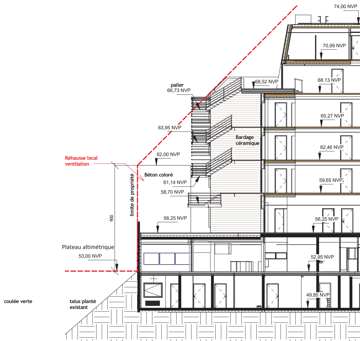
1 PCM2 Coupe sur prospect coulée verte 1 : 200
