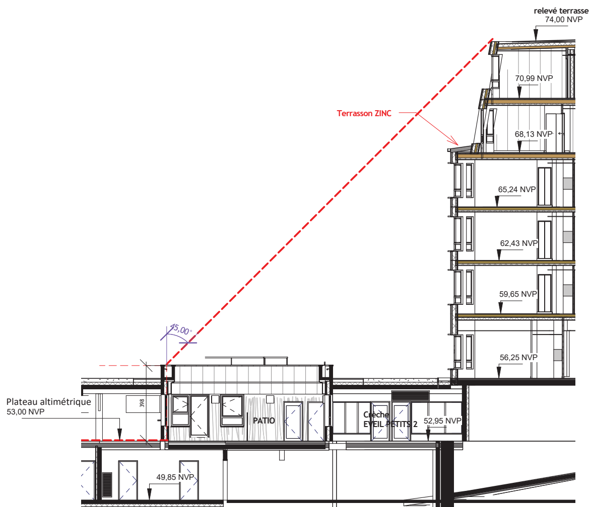
1 PCM2 Prospect immeuble voisin R+6 1 : 200
