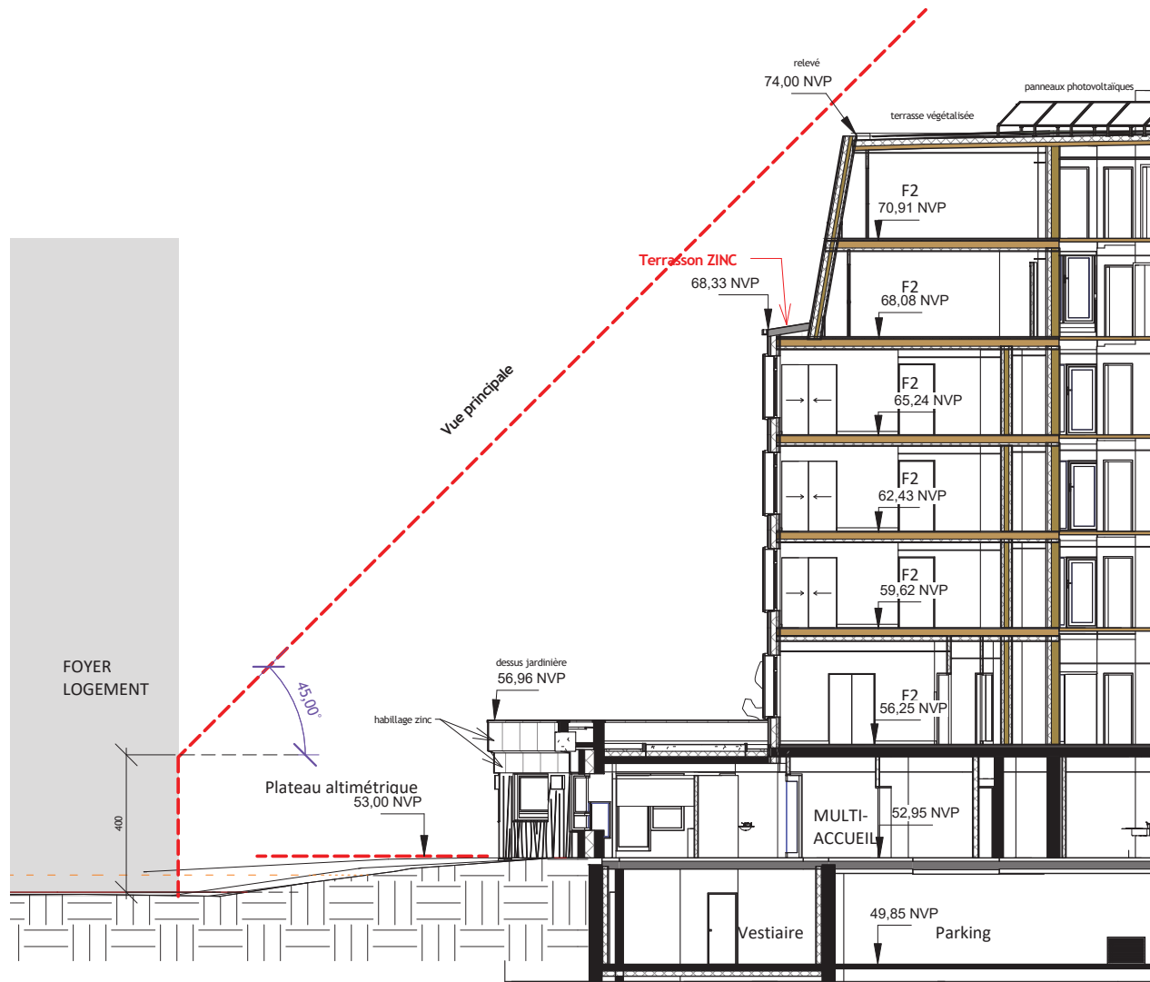
2 PCM2 Prospect vis à vis du foyer logement'
