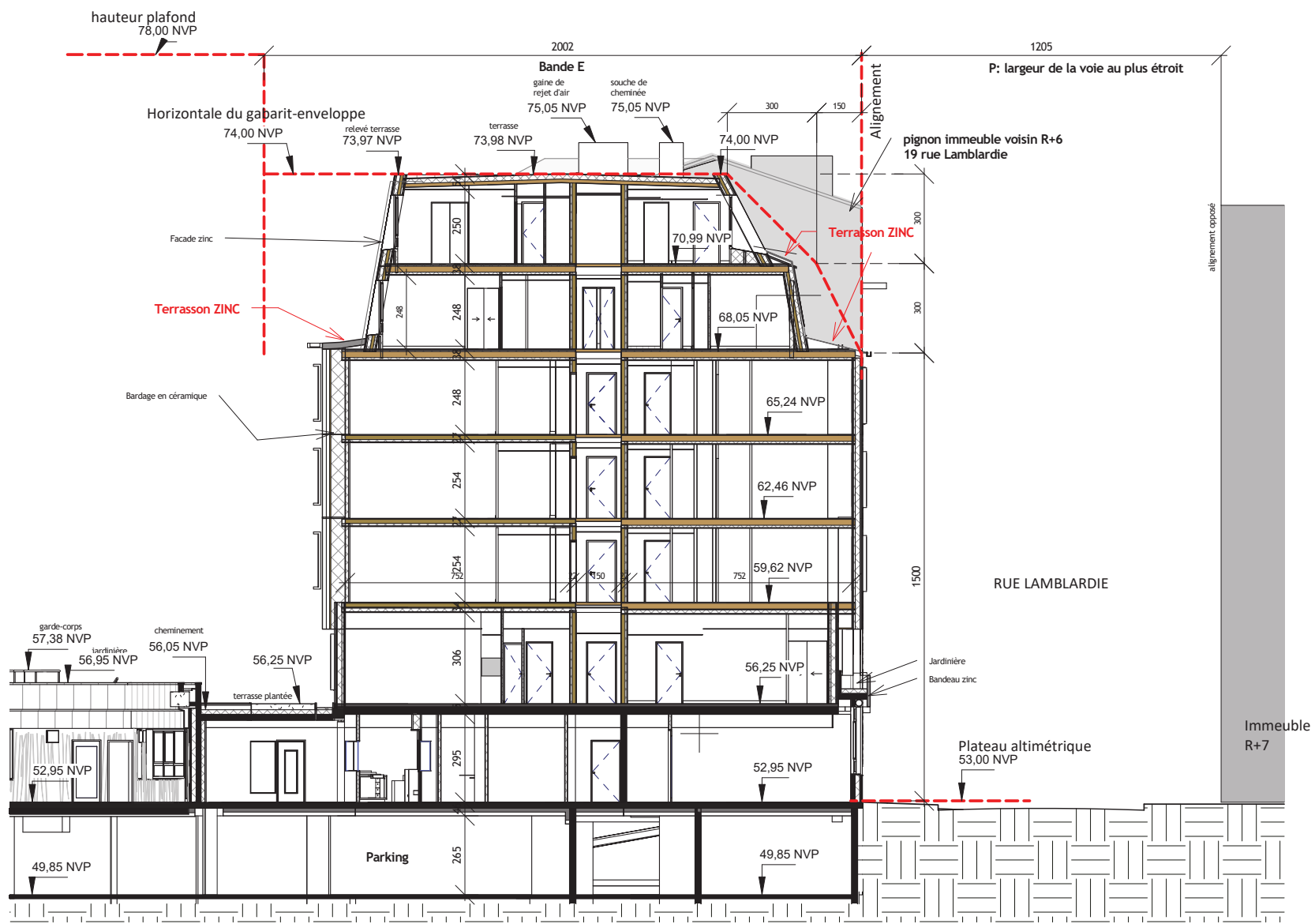
1 PCM2 Coupe sur rue Lamblardie Ech : 1 : 200
