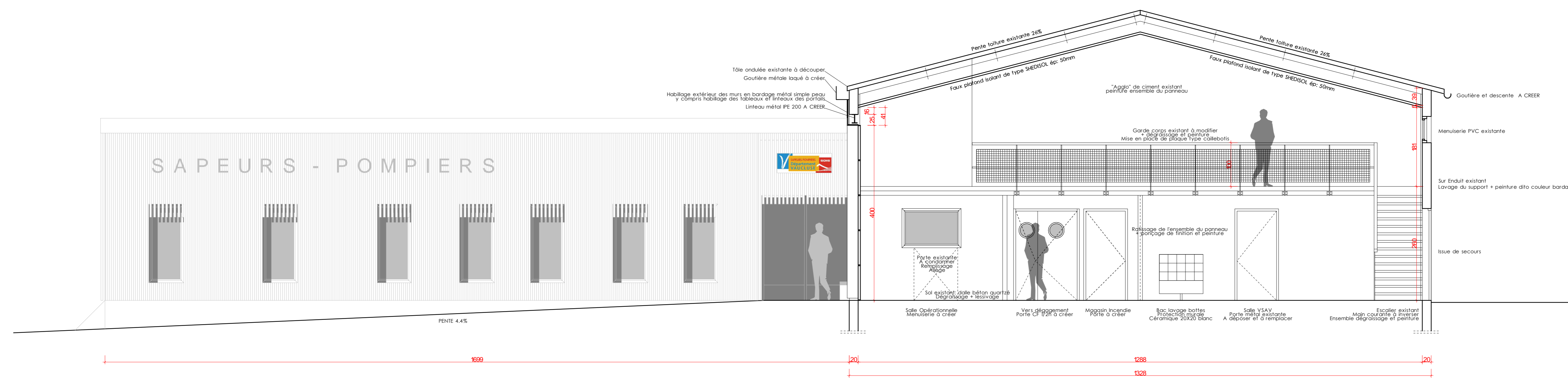
COUPE C
