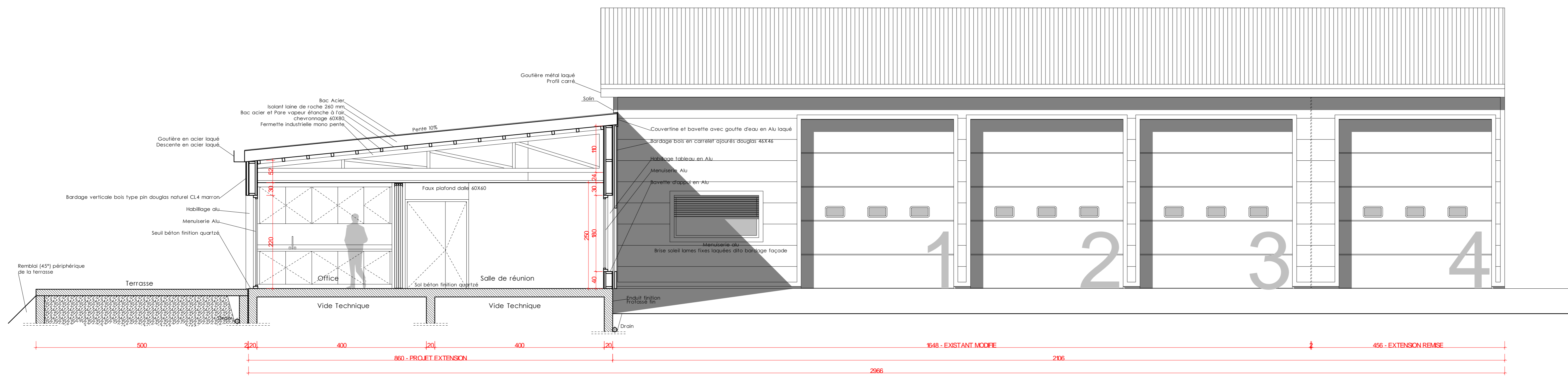
COUPE A
