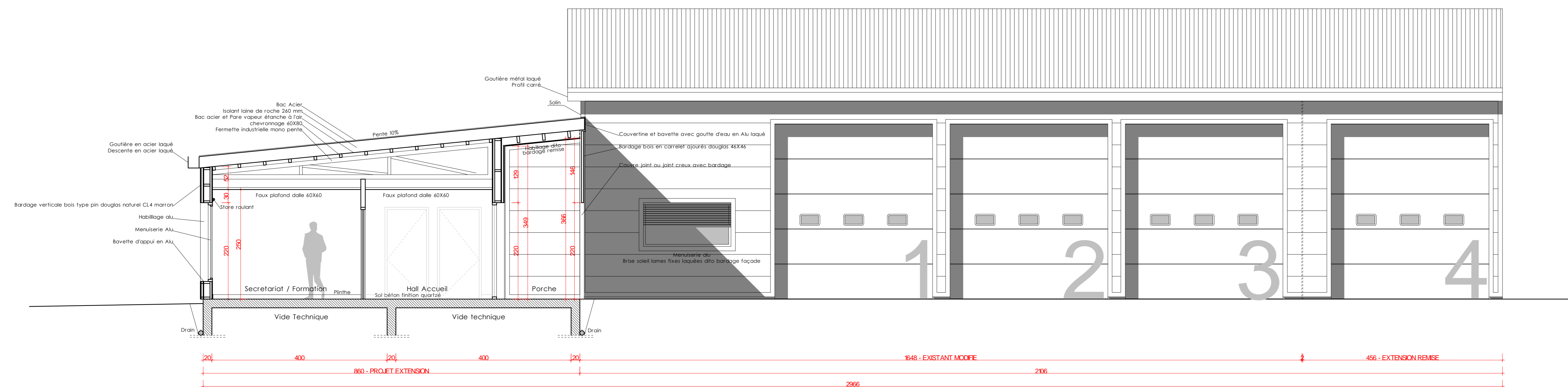
COUPE B
