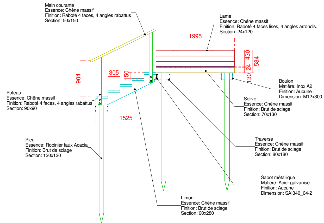
Vue de gauche
