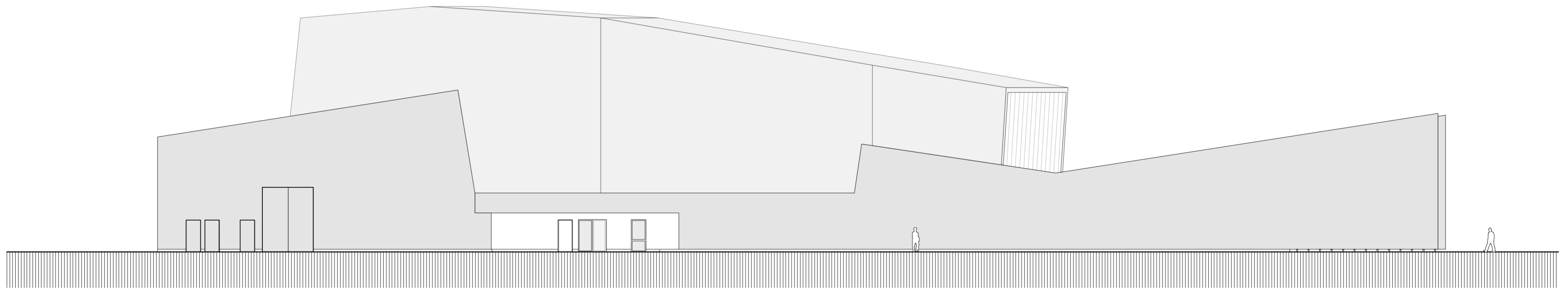
élévation Sud-Est
