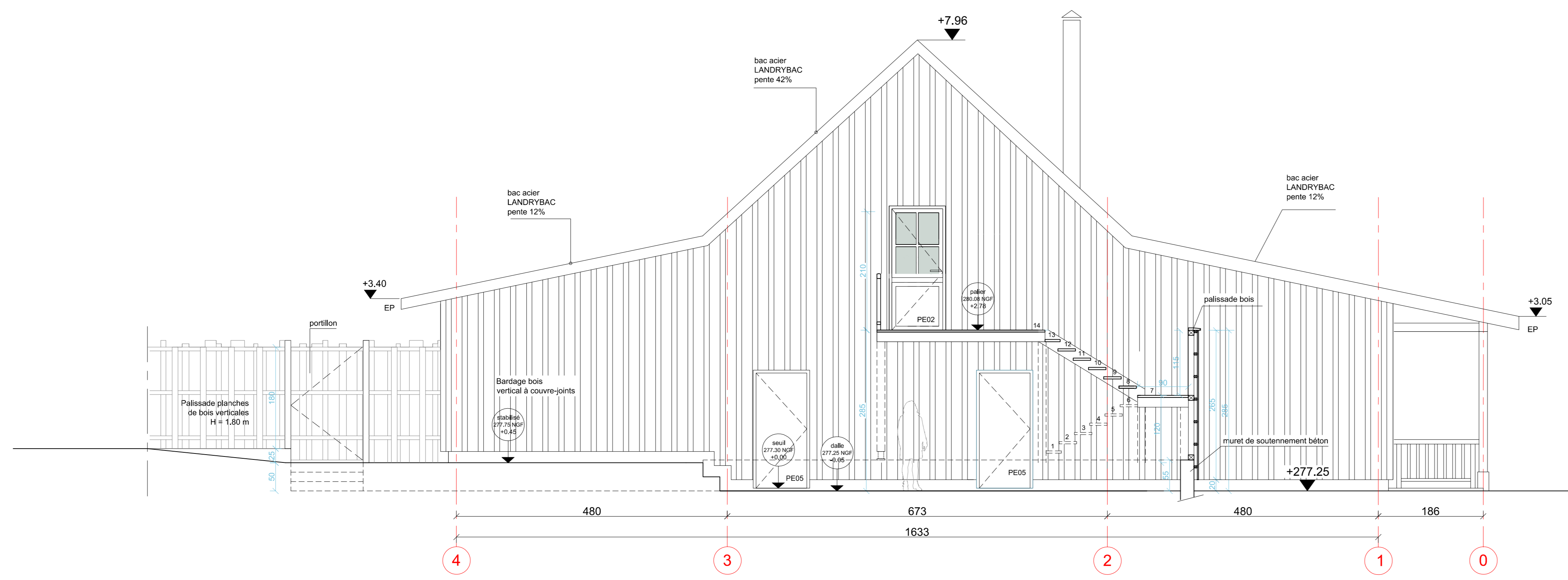
FAÇADE SUD EST niveau cour anglaise accès bâtiment d'Accueil 1/50e
