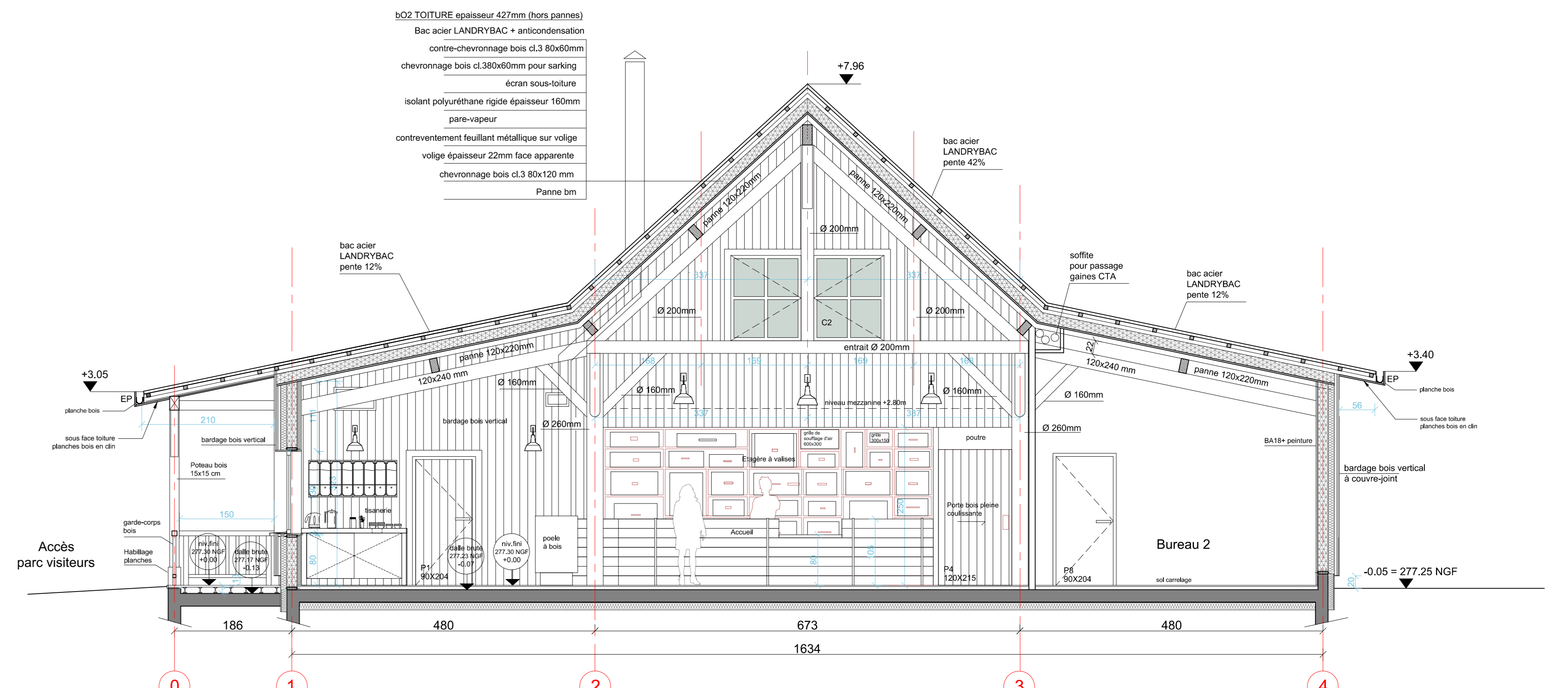
COUPE A-A Élévation portique file B 1/50e
