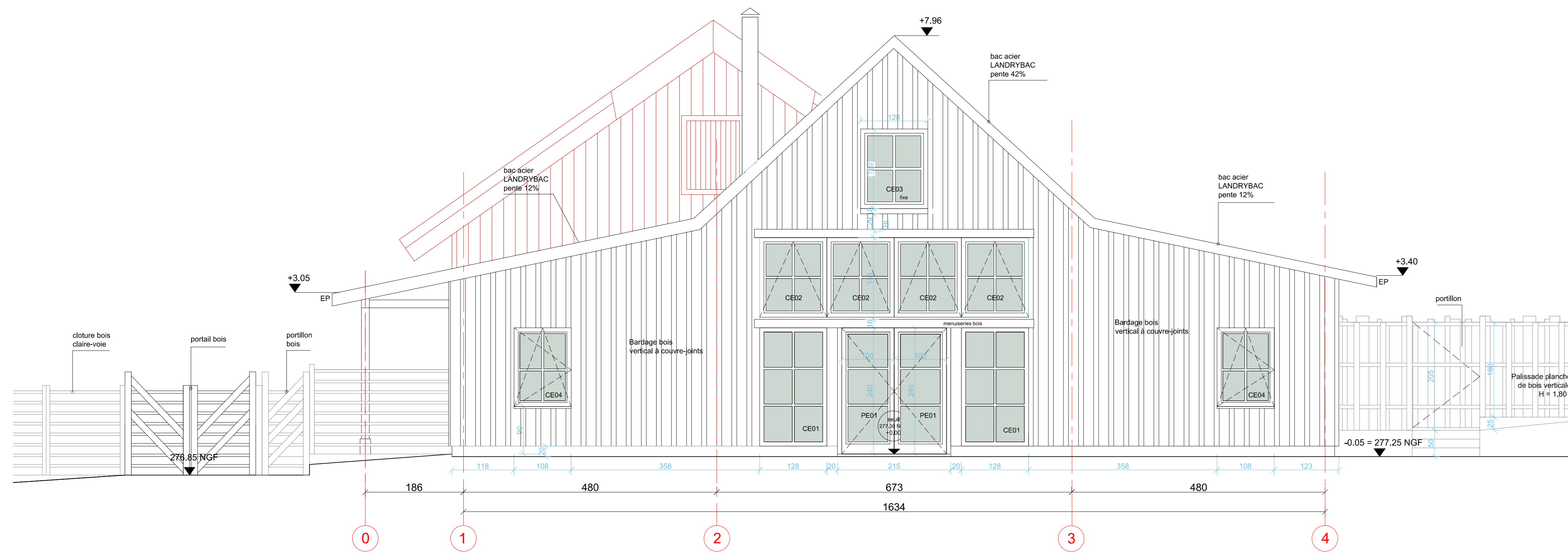
FAÇADE NORD OUEST 1/50e
