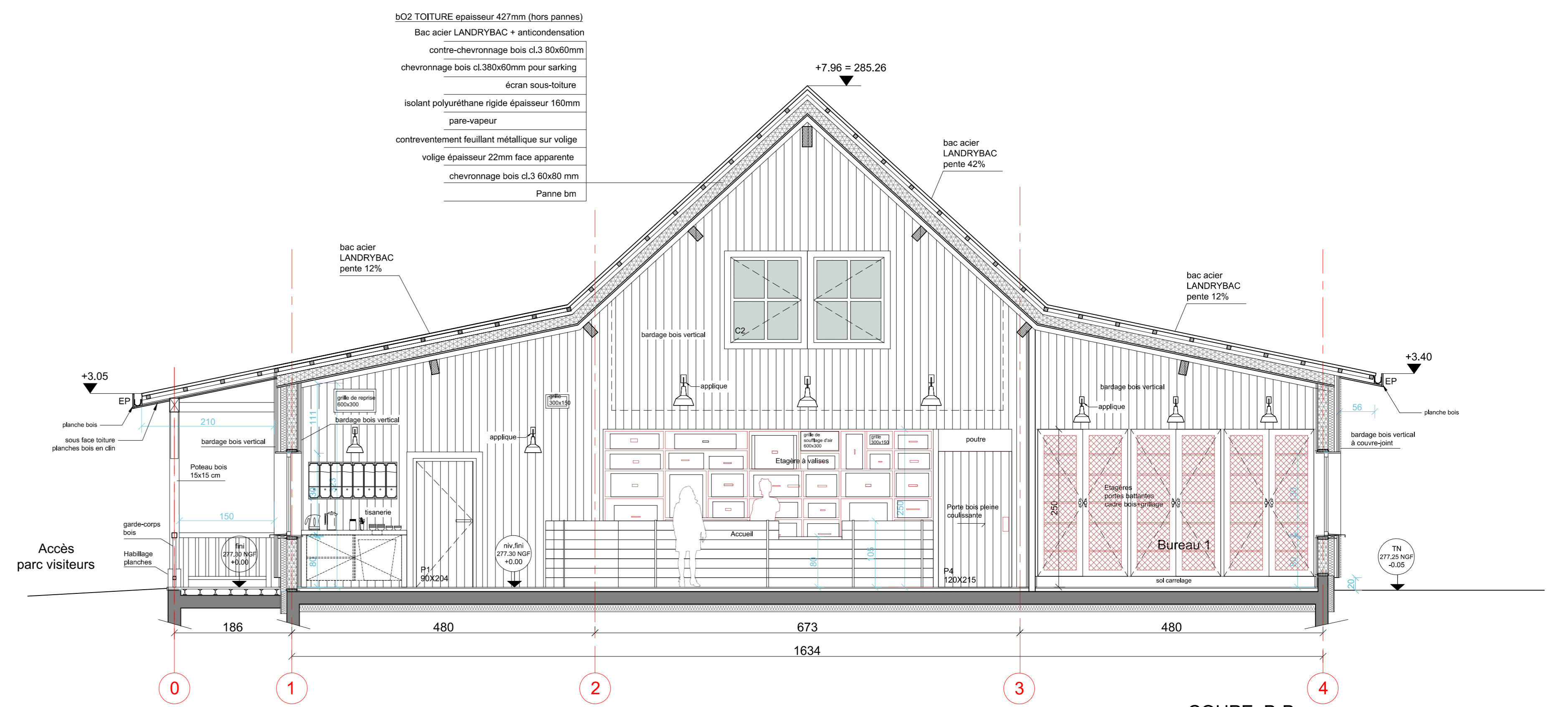
COUPE B-B 1/50e
