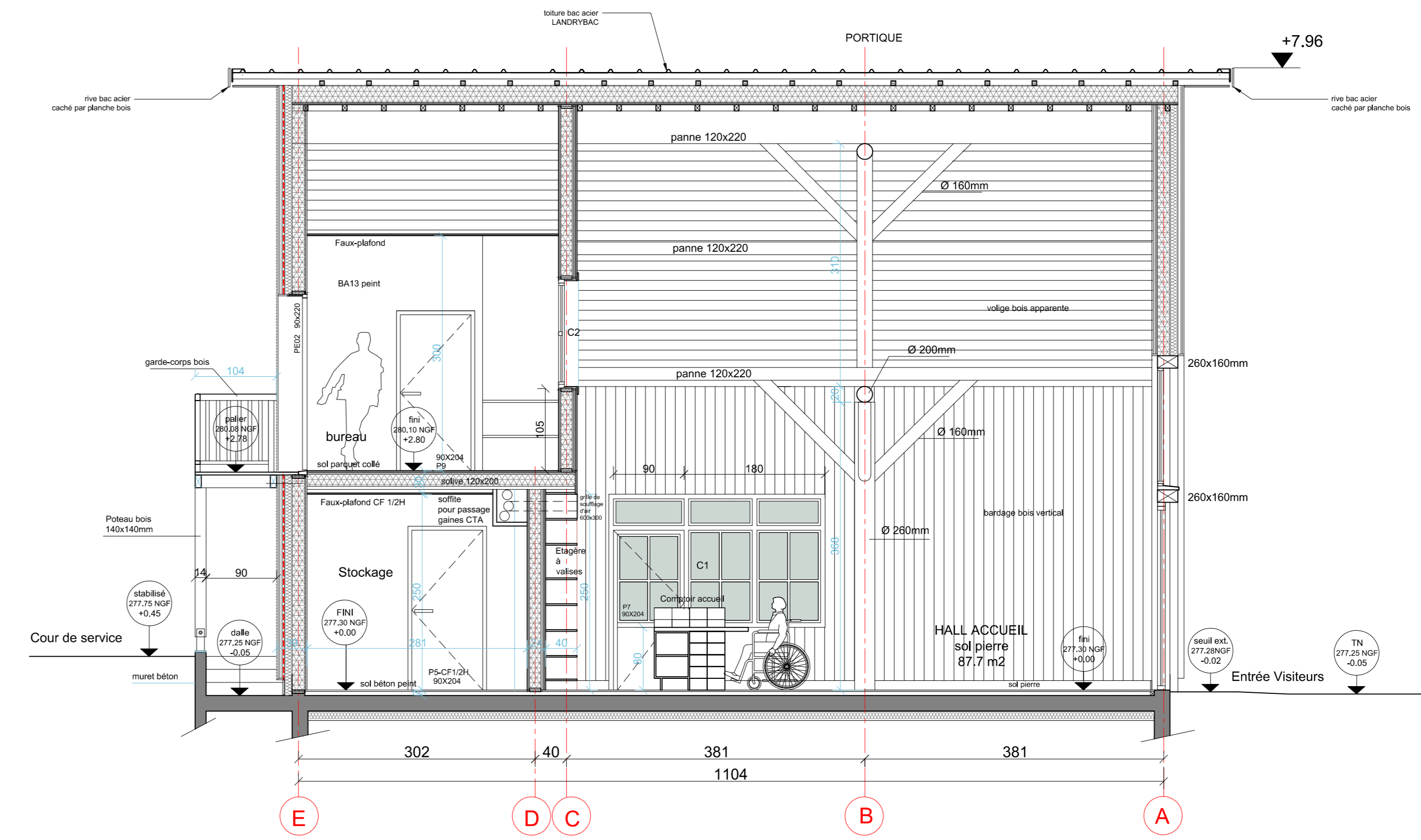
COUPE C-C 1/50e
