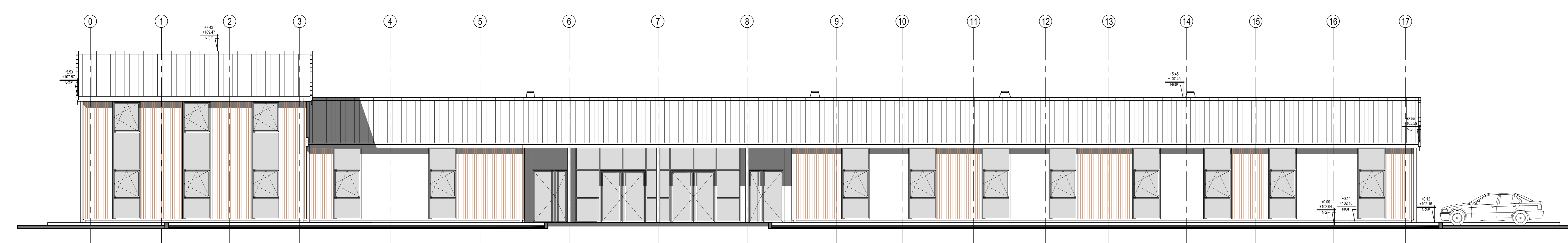
FAÇADE SUD OUEST - ETAT ACTUEL Ech. : 1/75
