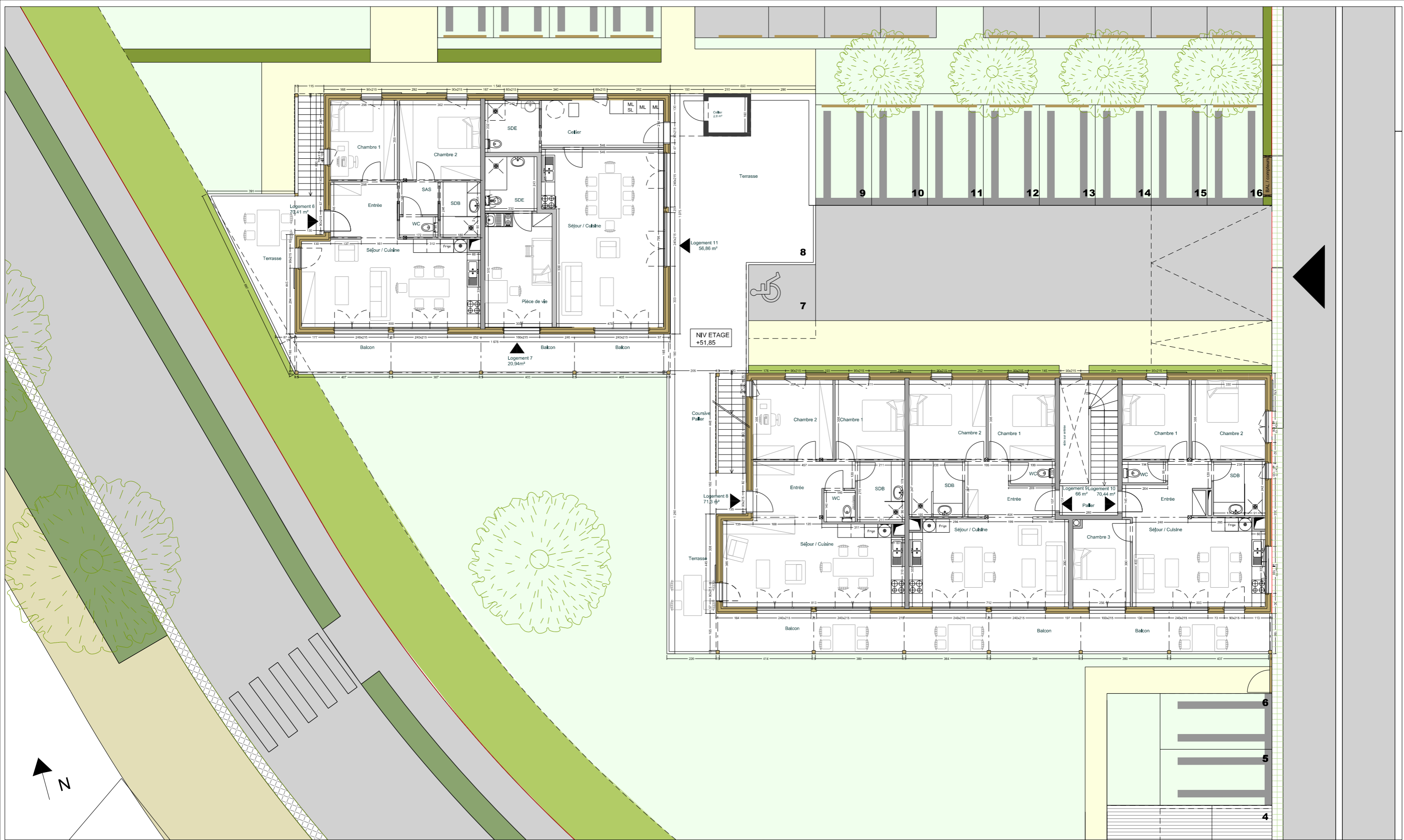
PLAN 1er étage - 1/150
