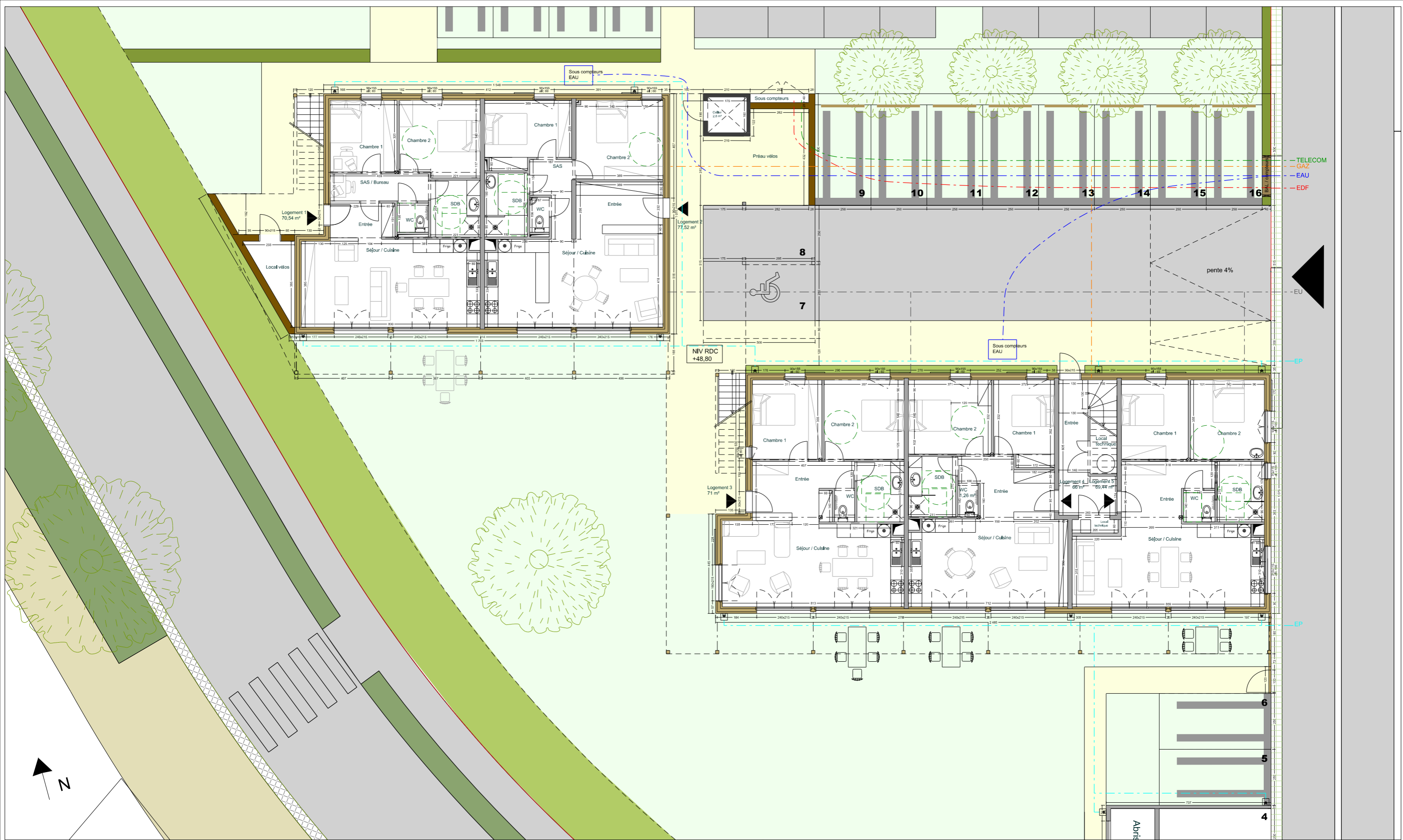
PLAN RDC - 1/150
