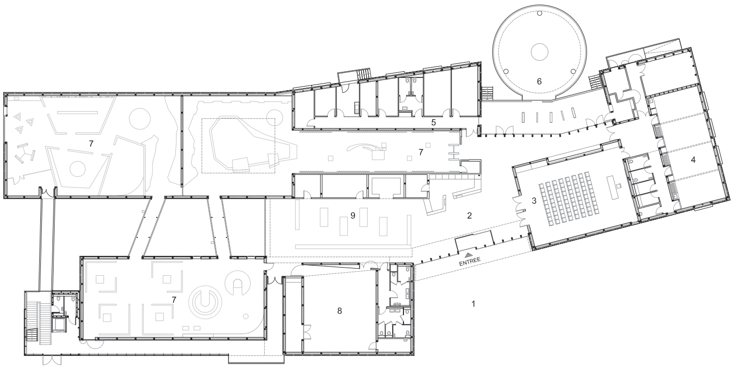
PLAN RDC
