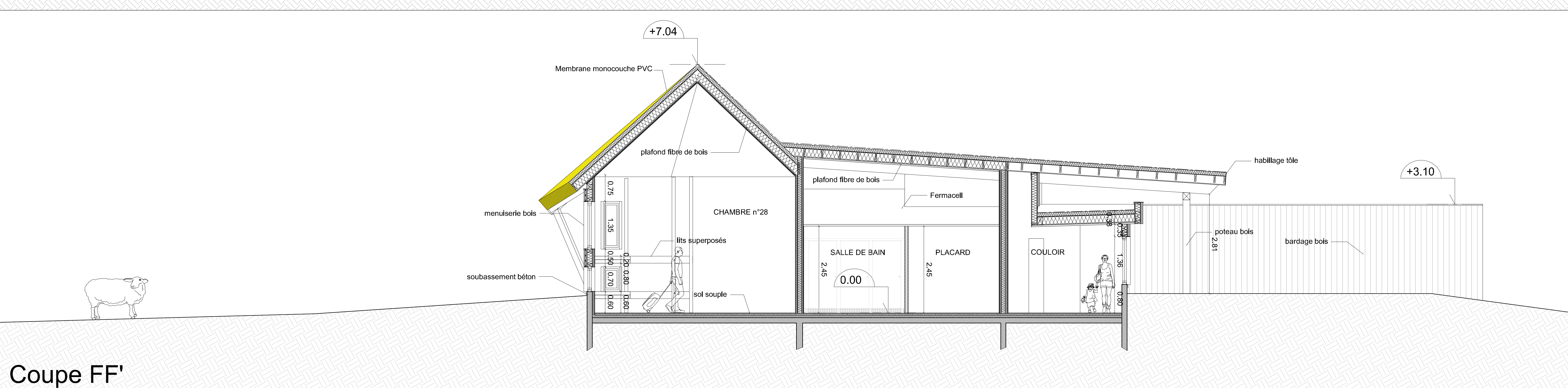
Coupe JJ'
