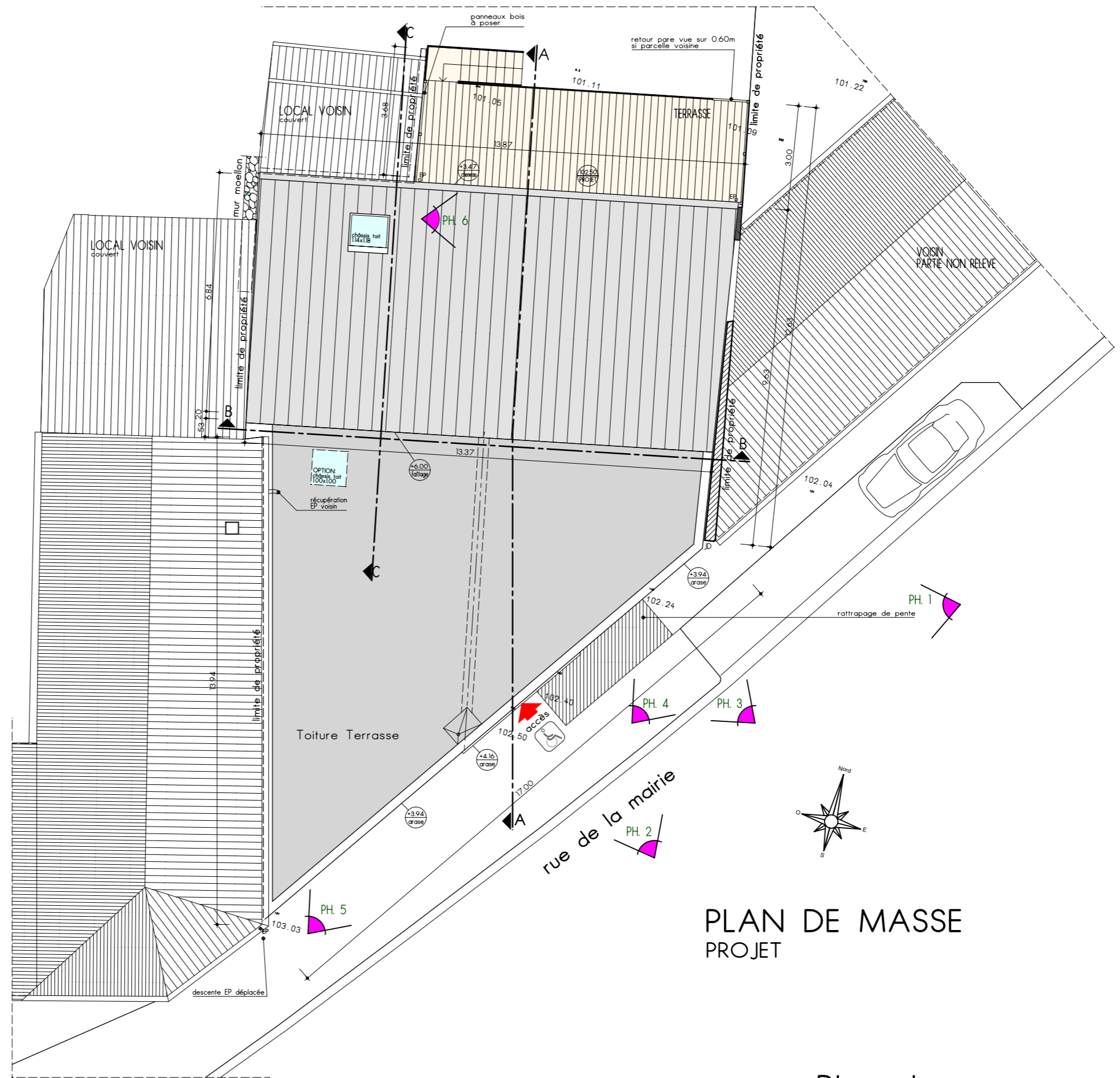
Plan de masse et des toitures Ech: 1/125
