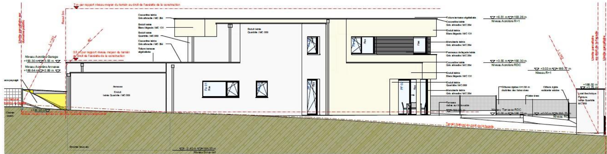
Façade NordOuest
