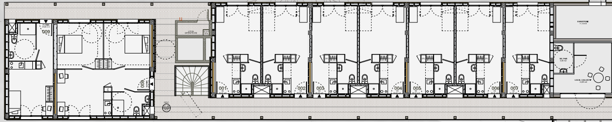
PLAN DU REZ-DE-CHAUSSÉE
