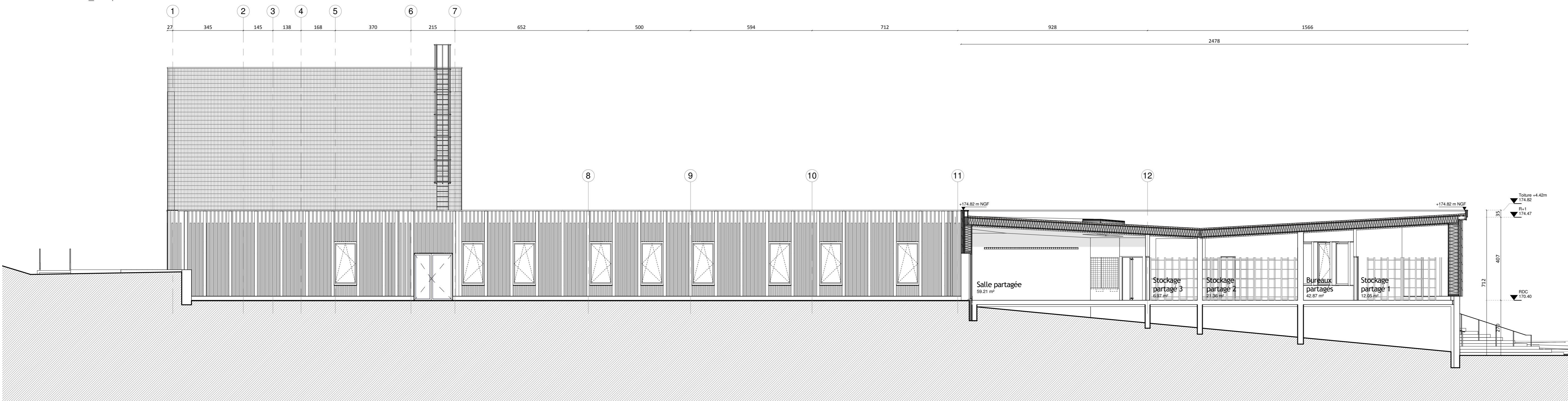
Ech : 1 : 100 COU_Coupe détail 07
