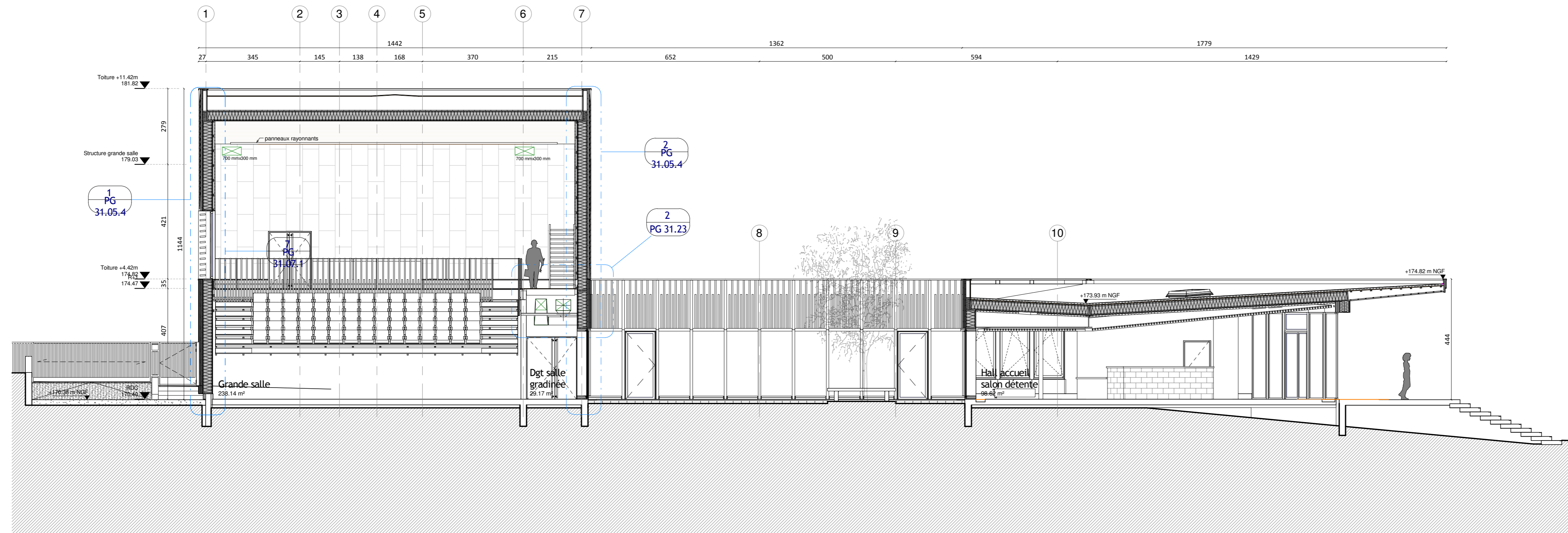
Ech : 1 : 100 COU_Coupe détail 03
