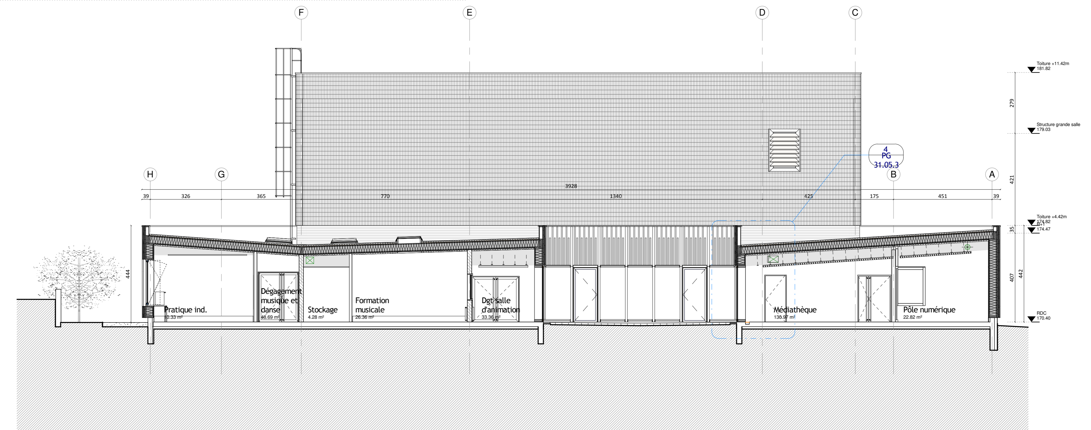
Ech : 1 : 100 COU_Coupe détail 09
