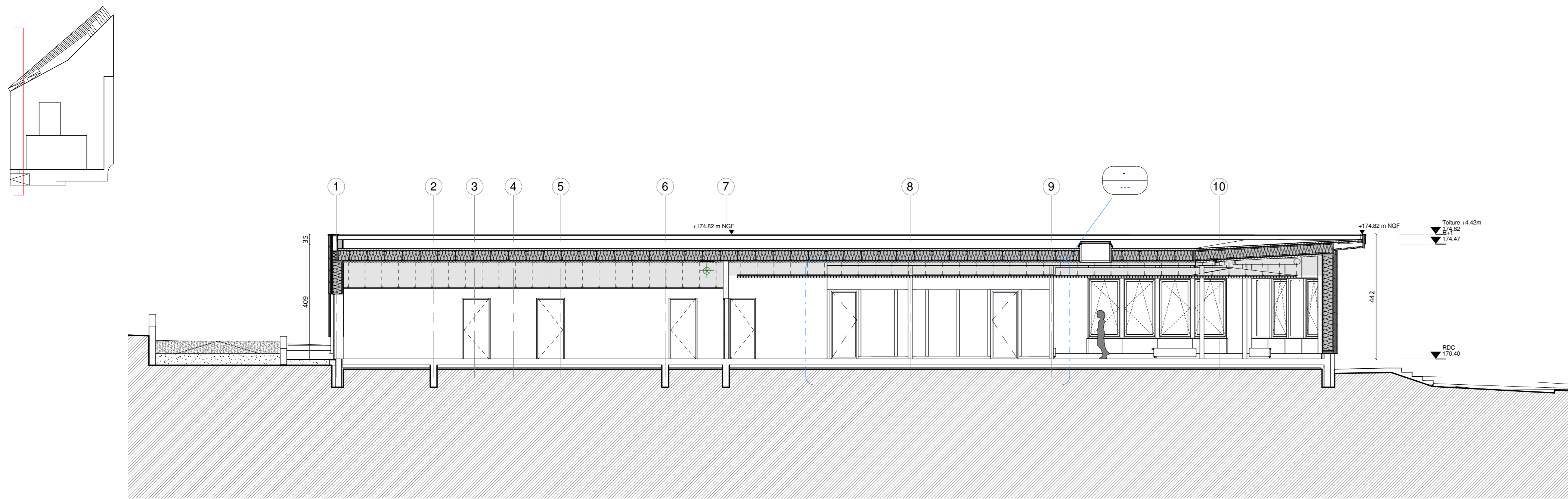
Ech : 1 : 100 COU_Coupe détail 01
