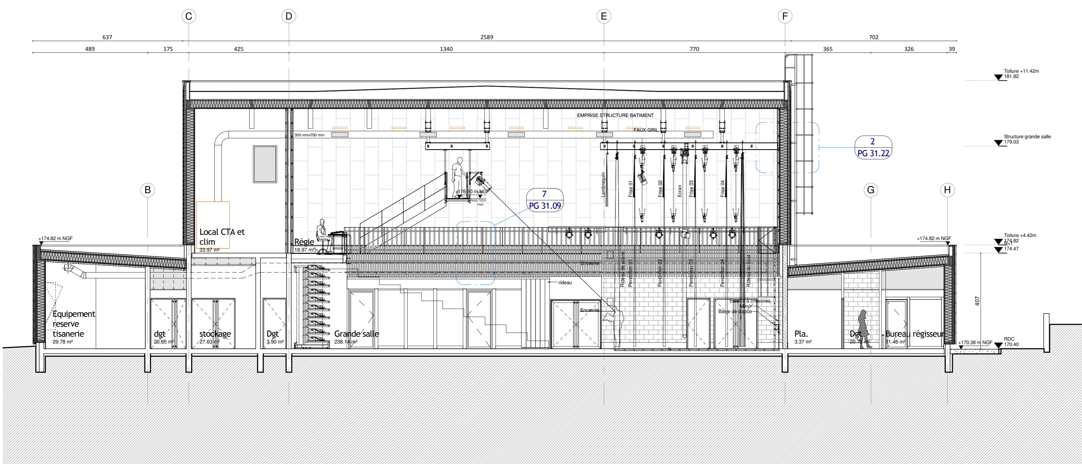
Ech : 1 : 100 COU_Coupe détail 10
