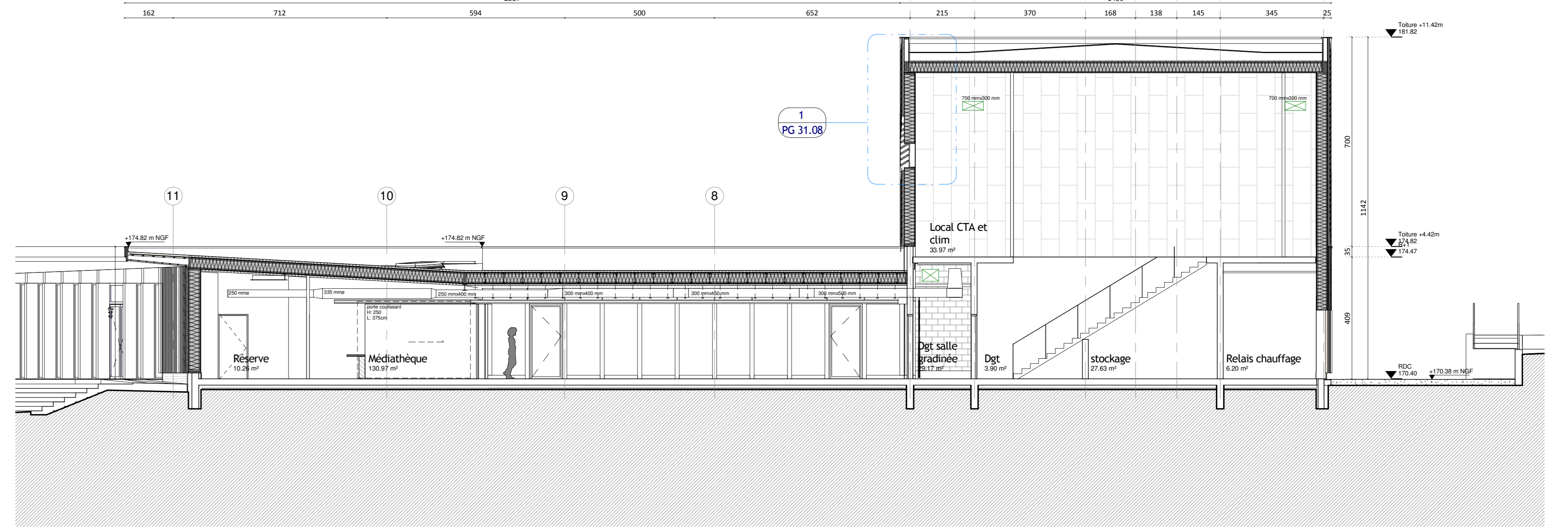
Ech : 1 : 100 COU_Coupe détail 02
