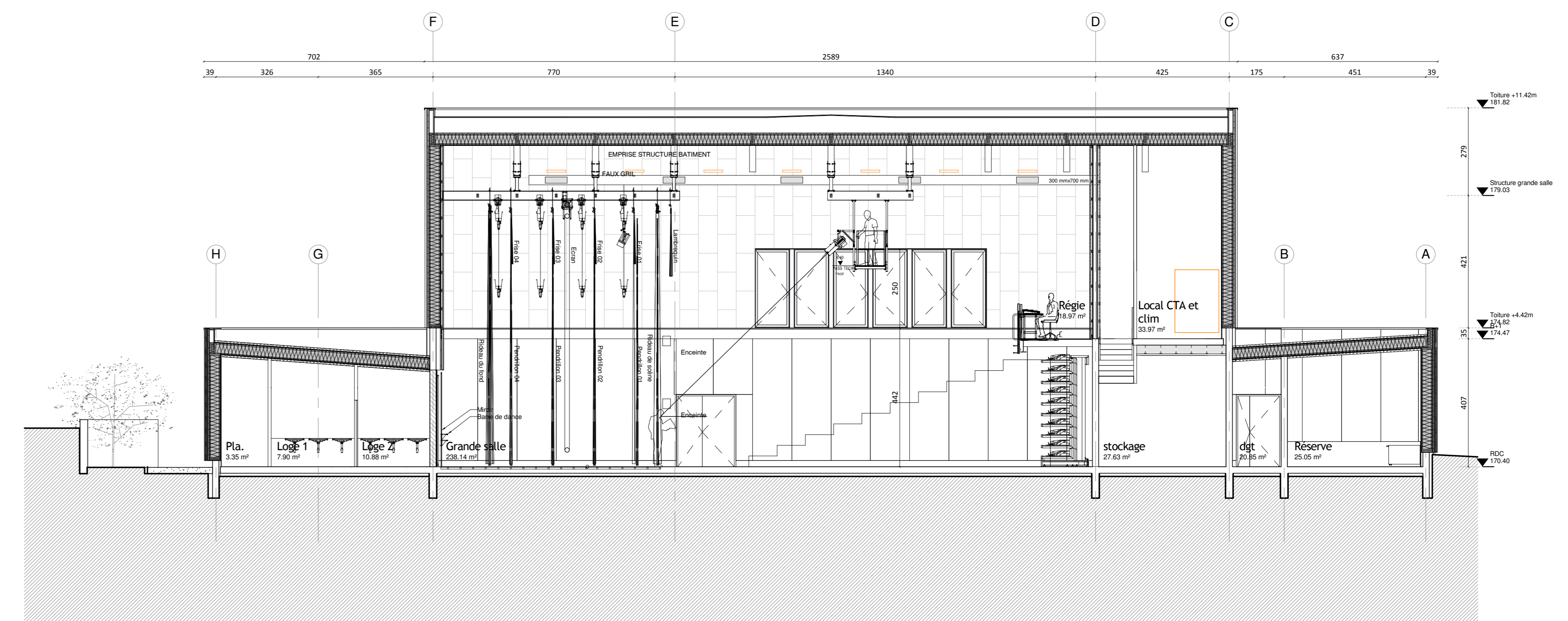
Ech : 1 : 100 COU_Coupe détail 11
