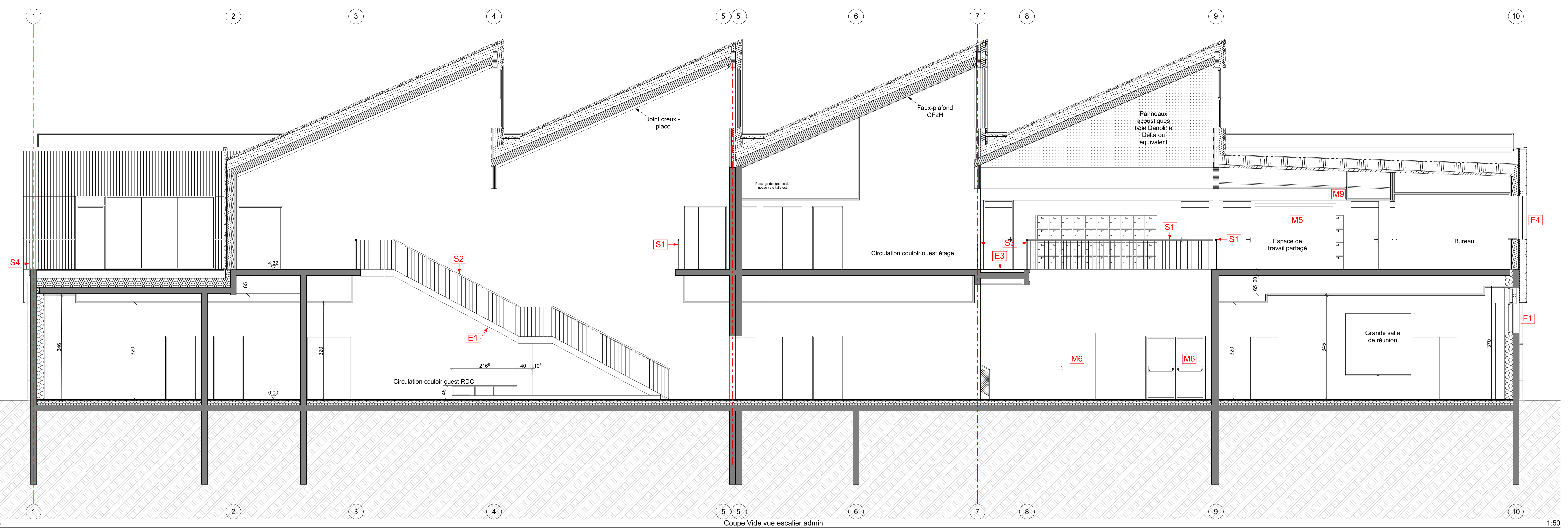
Coupe Vide vue escalier admin
