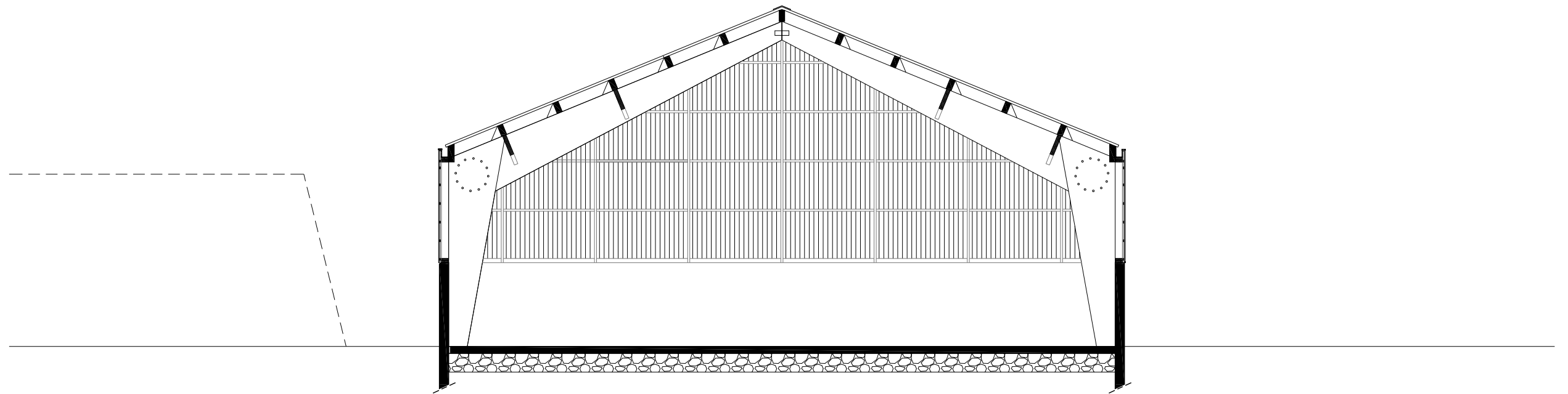
0 0,5 1 2 COUPE BB
